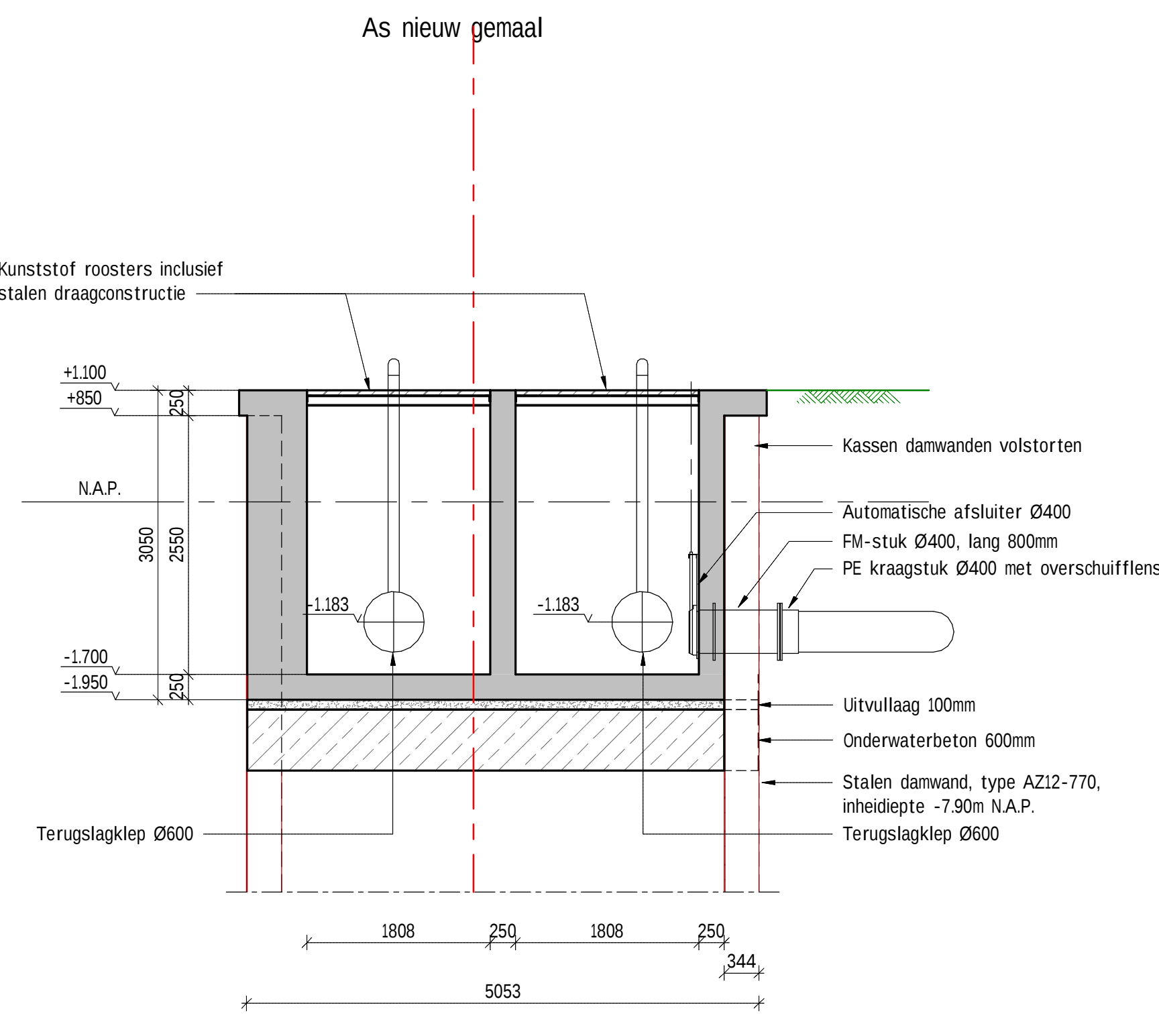
Doorsnede C-C
