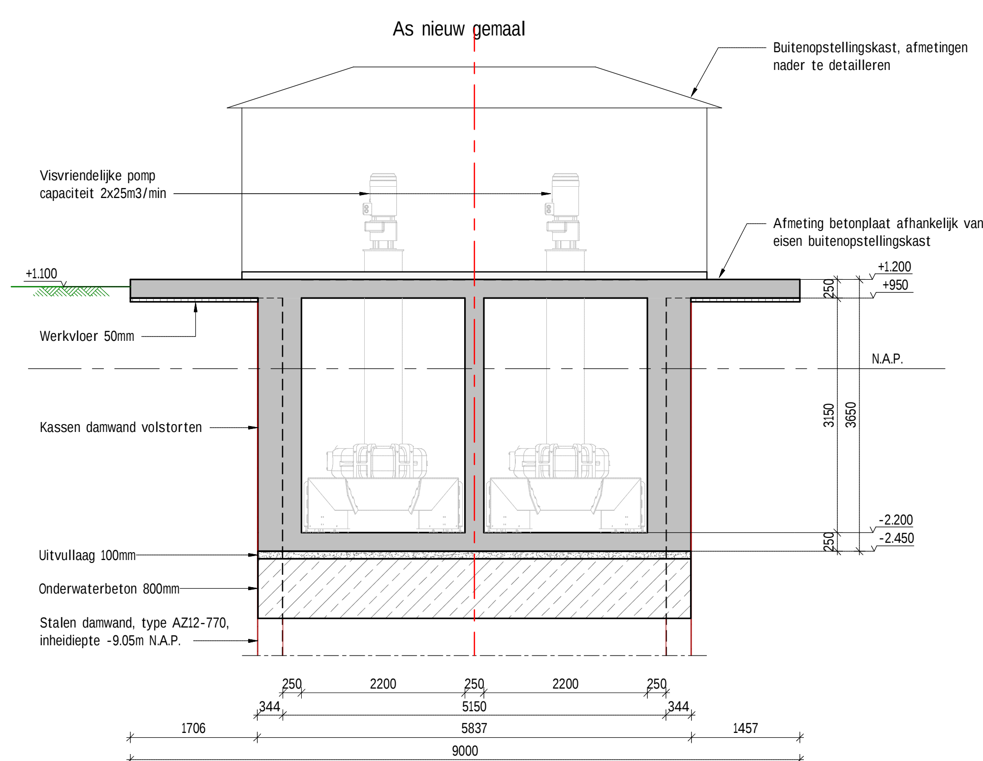
Doorsnede B-B
