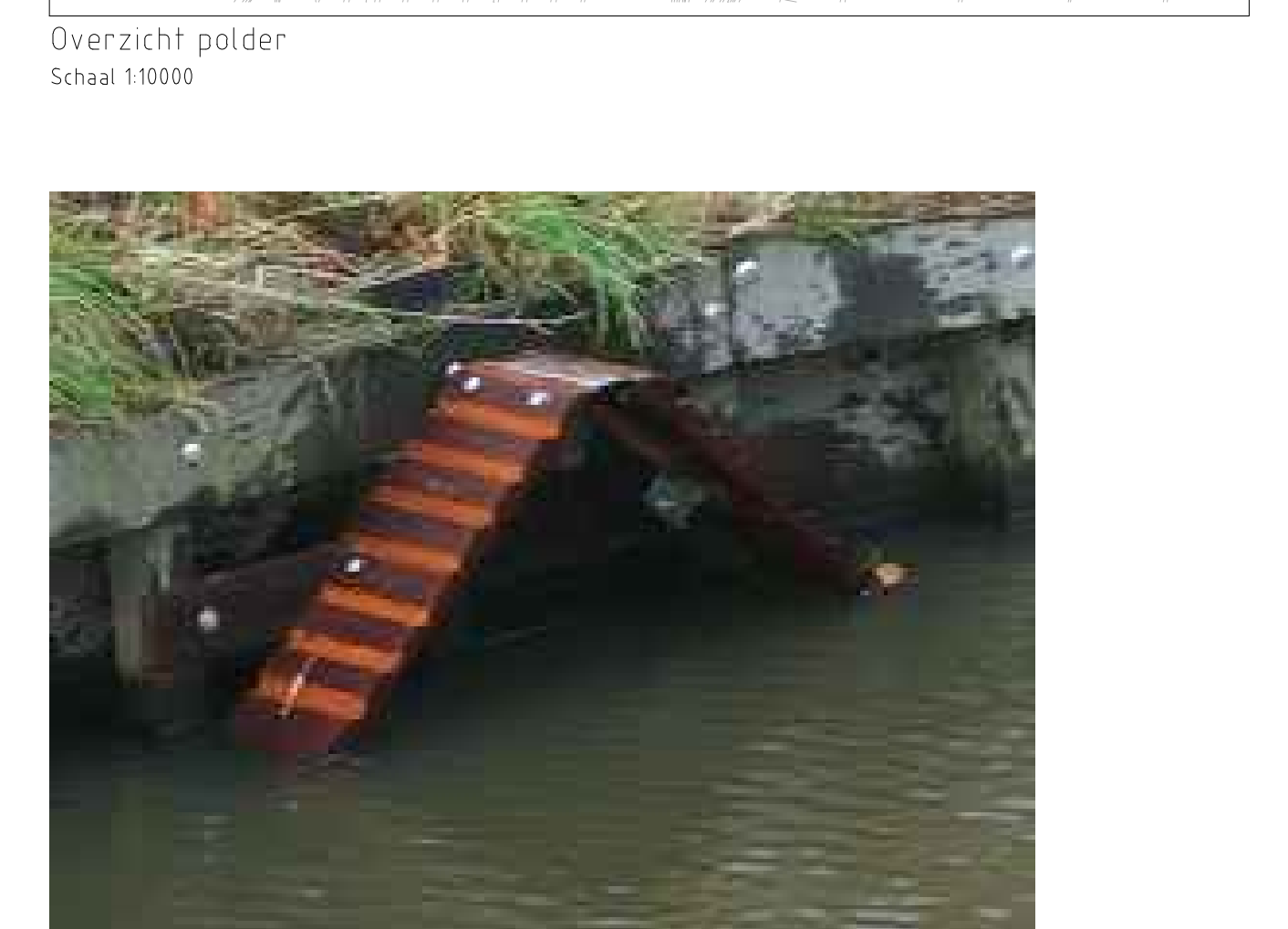
Principe detail A: Fauna uitrede plaats
