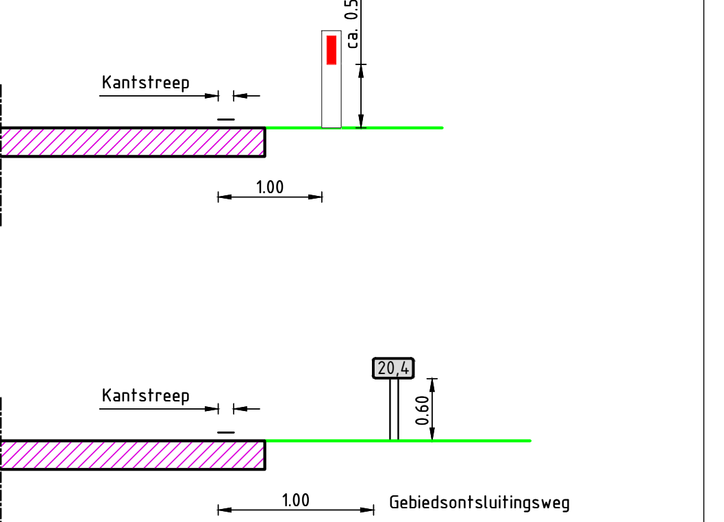
Detail 34 Plaatsing hectometerborden en reflectoren SCHAAL 1:50
