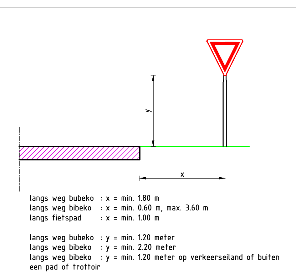
Detail 30 Plaatsing flespalen verkeersborden SCHAAL 1:50
