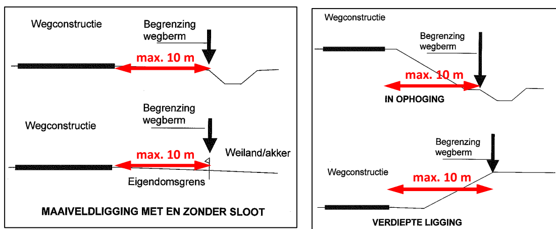
Figuur 4.2: Begrenzing bermen
