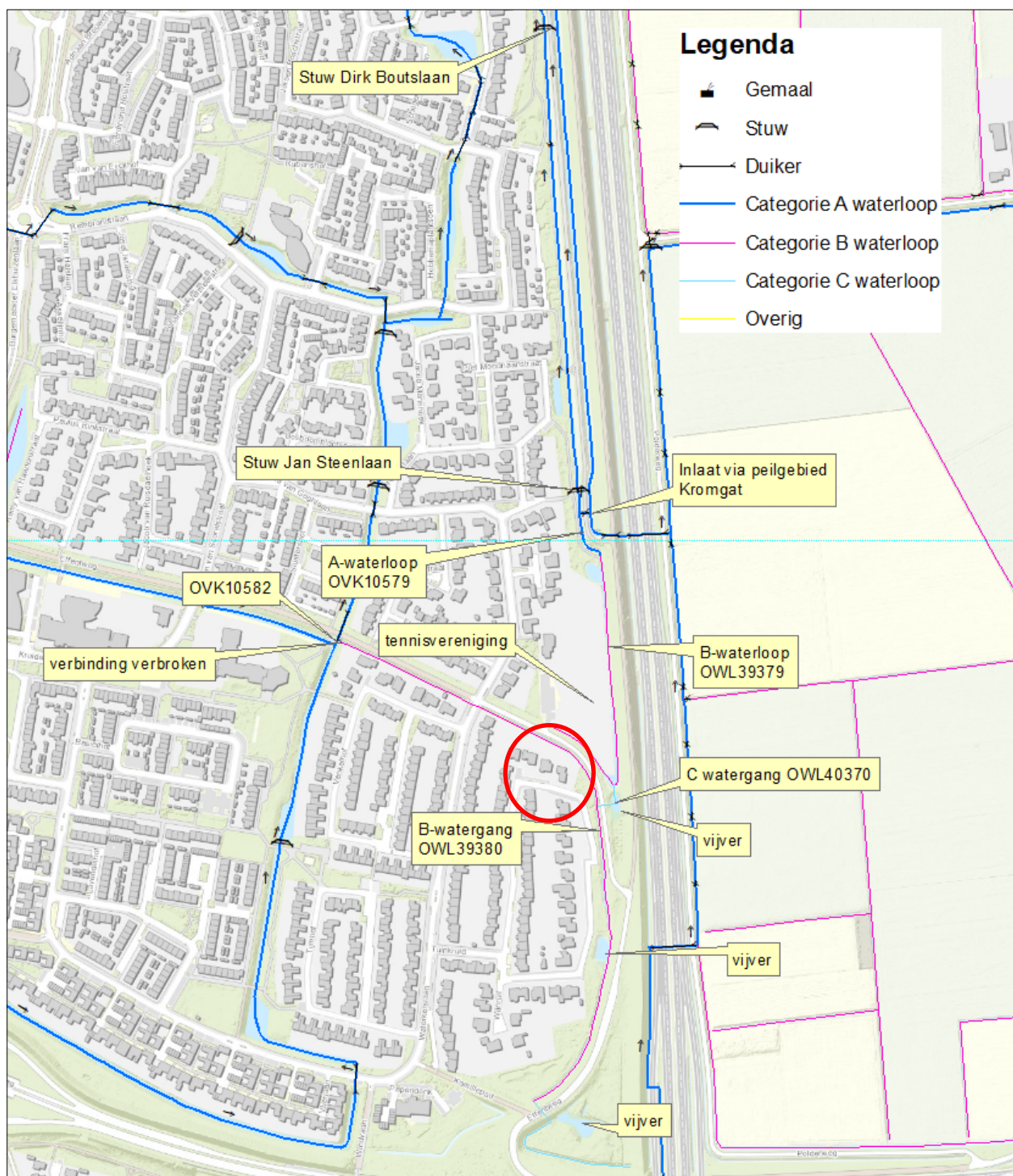
Figuur 1 Situatieschets waterhuishouding in de wijk Dommelbergen te Oosterhout
