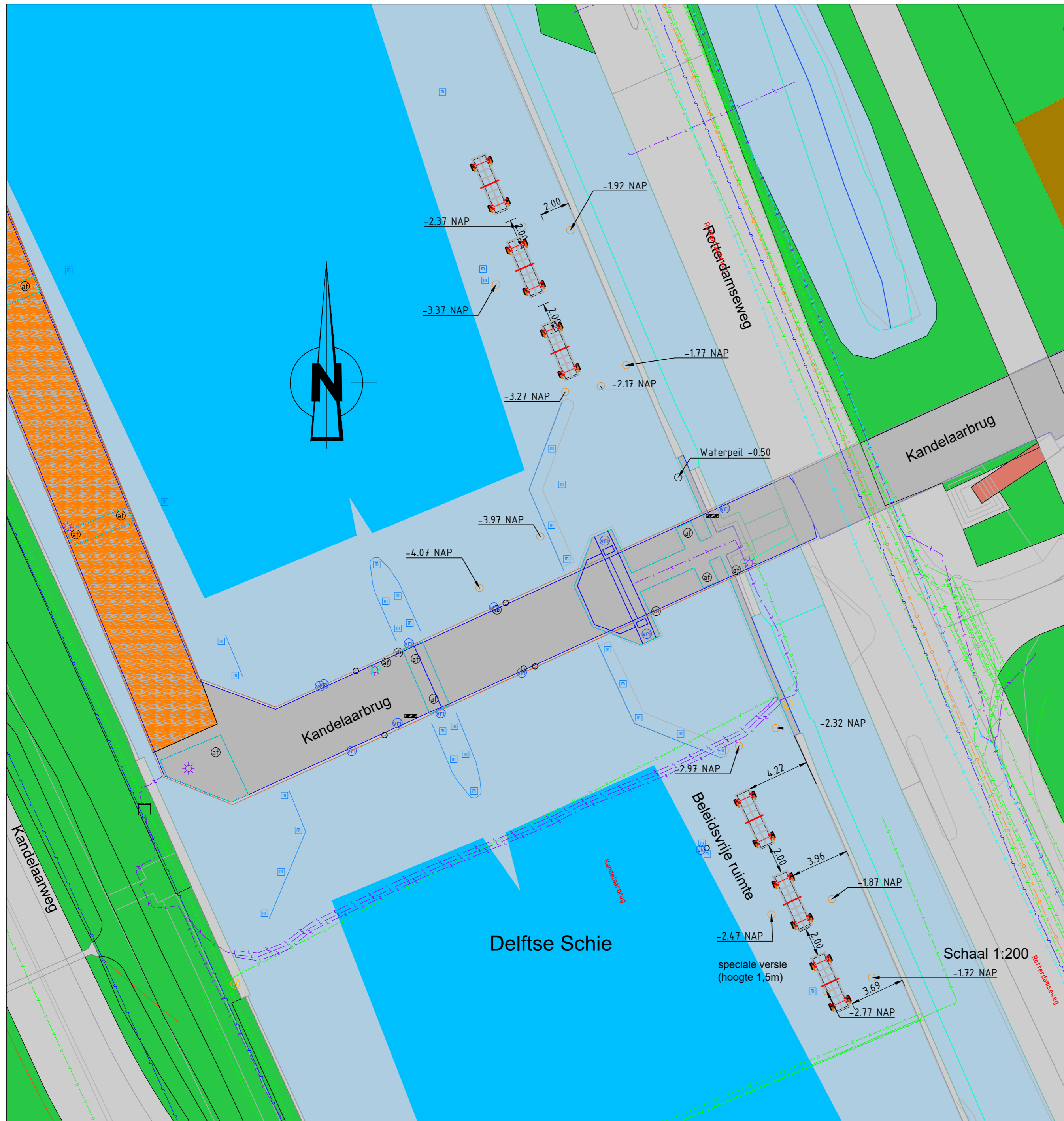
Situatie SCHAAL 1 : 200
