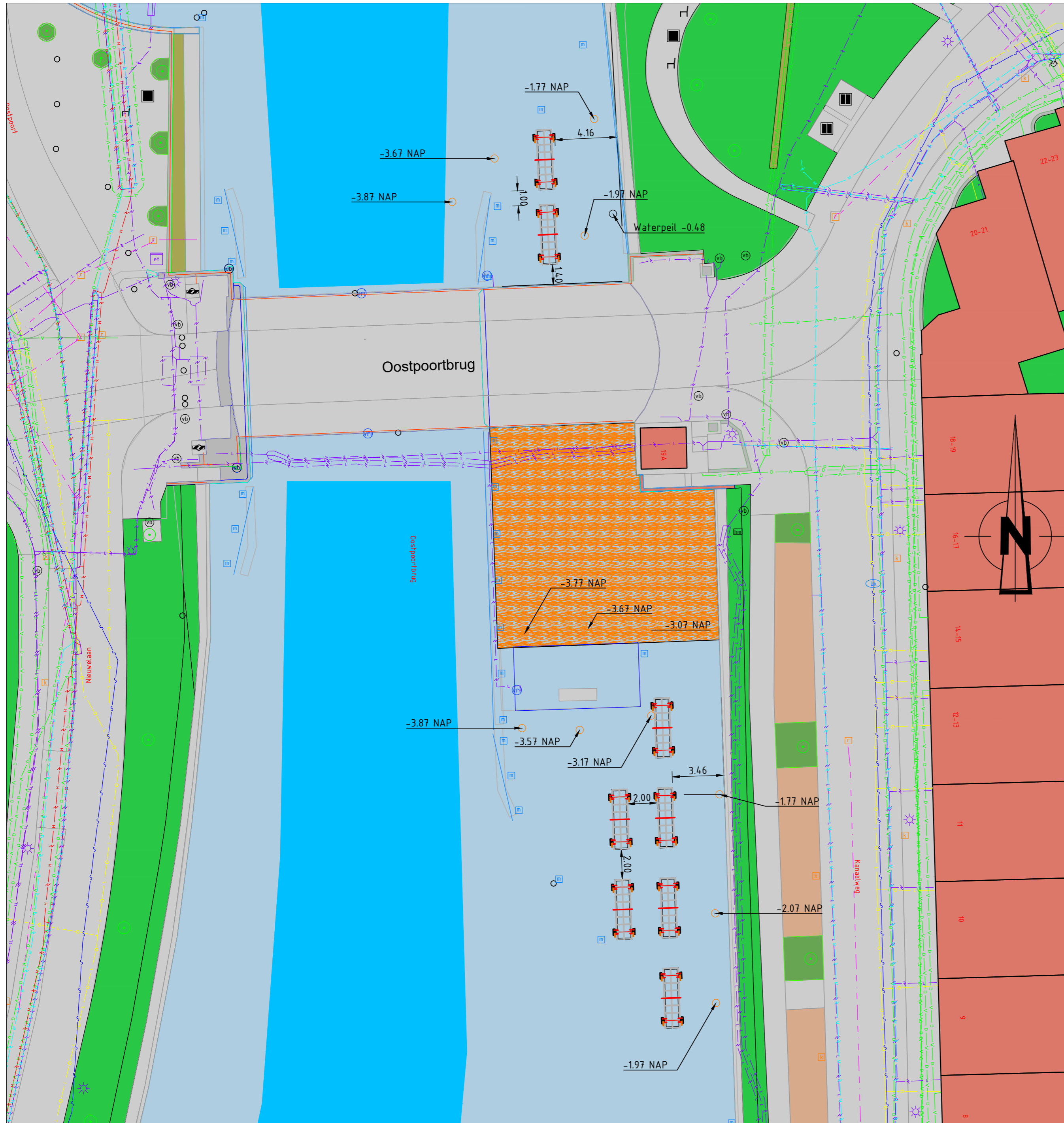
Situatie SCHAAL 1 : 200
