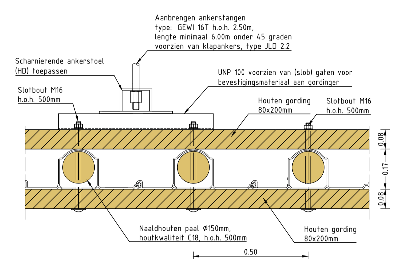
DETAIL B PROLOCK DAMWAND Schaal 1:10 bovenaanzicht
