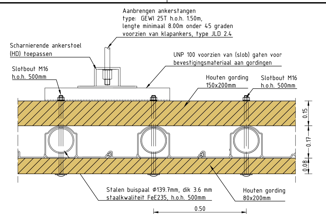
DETAIL A PROLOCK DAMWAND Schaal 1:10 bovenaanzicht
