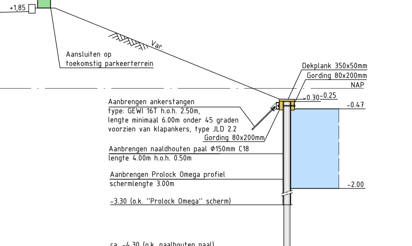
PRINCIPEDOORSNEDE B PROLOCK DAMWAND Schaal 1:50 doorsnede
