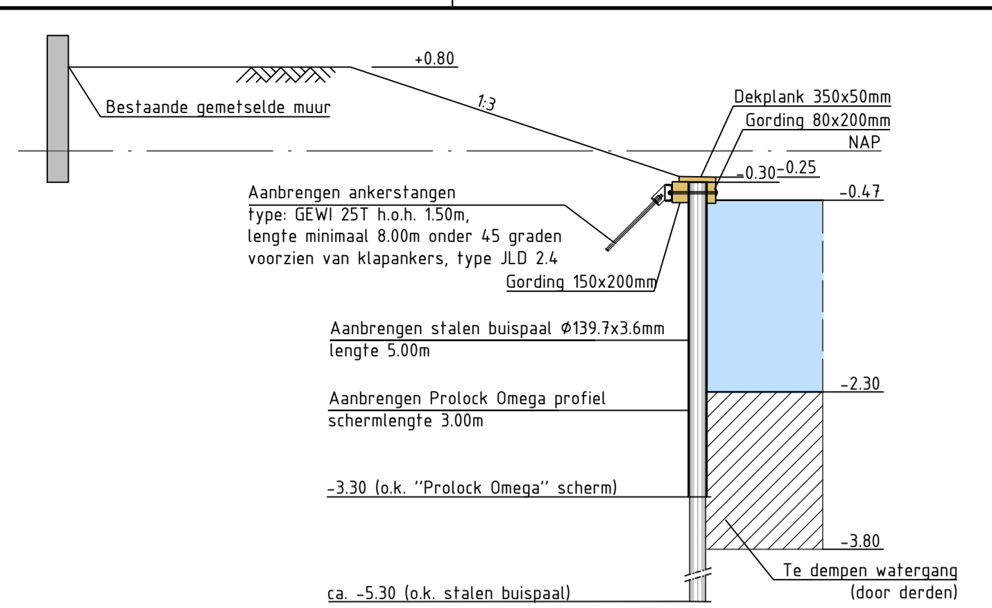
PRINCIPEDOORSNEDE A PROLOCK DAMWAND Schaal 1:50 doorsnede
