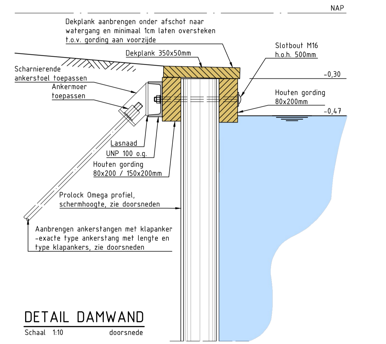
DETAIL DAMWAND Schaal 1:10 doorsnede
