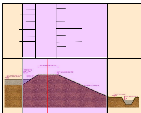
AFBEELDING 19.6 OVERZICHT LEGGERZONES WATERKERINGEN
