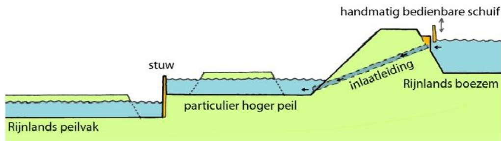
AFBEELDING 17.1 WATERINLAAT DOOR EEN WATERKERING
