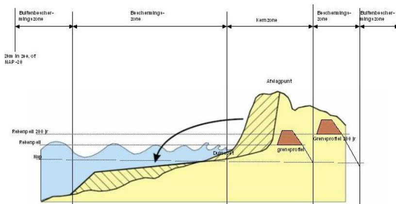
AFBEELDING 20.6 GRENSPROFIEL ZEEWERING
