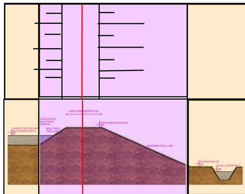
AFBEELDING 19.7 OVERZICHT LEGGERZONES WATERKERINGEN
