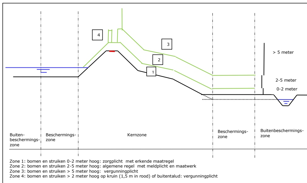
AFBEELDING 23.1 ZONERING VOOR NIEUWE BEPLANTING OP WATERKERINGEN
