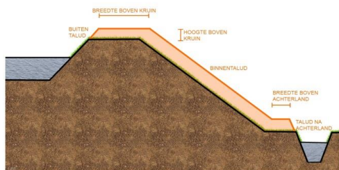
AFBEELDING 25.4 PROFIEL VAN VRIJE RUIMTE (ORANJE LIJN)
