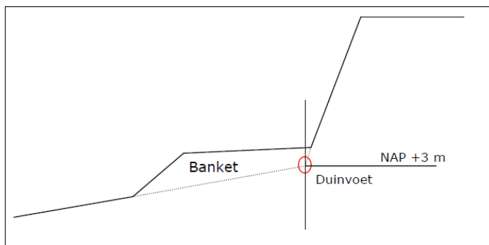
AFBEELDING 19.5 LIGGING DUINVOET
