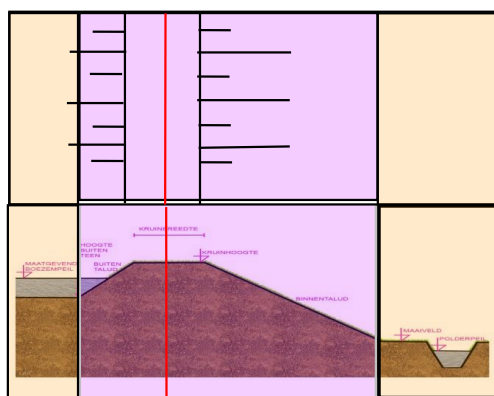
AFBEELDING 20.2 OVERZICHT LEGGERZONES WATERKERINGEN
