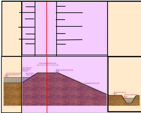
AFBEELDING 21.2 OVERZICHT LEGGERZONES WATERKERINGEN
