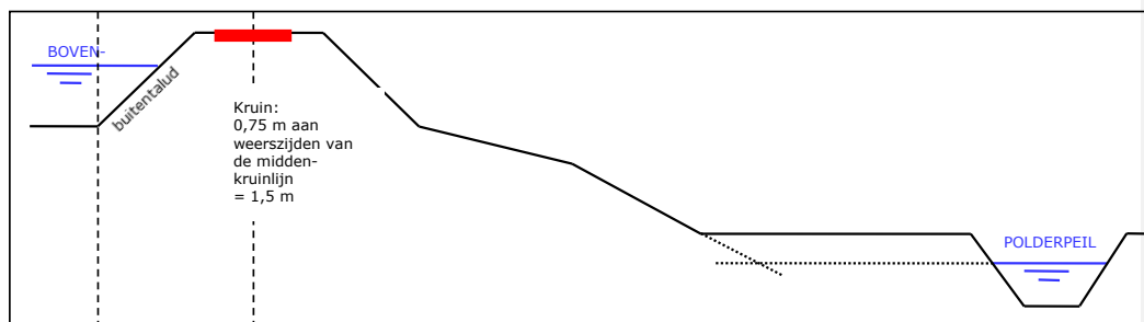
AFBEELDING 19.3 LIGGING VAN DE KRUIJN VAN DE WATERKERING
