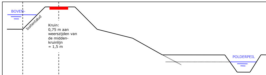
AFBEELDING 25.3 LIGGING VAN DE KRUIJN VAN DE WATERKERING
