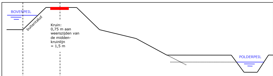
AFBEELDING 23.5 BUITENTALUD EN KRUIJN VAN DE WATERKERING
