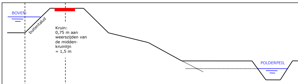
AFBEELDING 20.3 KRUIJN VAN DE WATERKERING
