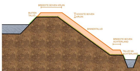
AFBEELDING 20.4 PROFIEL VAN VRIJE RUIMTE
