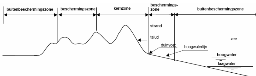
AFBEELDING 20.1 OVERZICHT LEGGERZONES ZEEWERING
