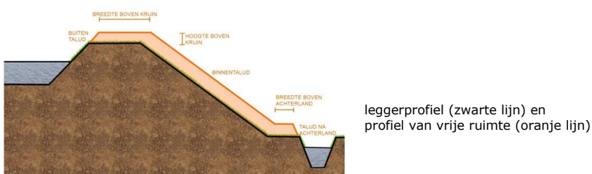
AFBEELDING 20.7 PROFIEL VAN VRIJE RUIMTE
