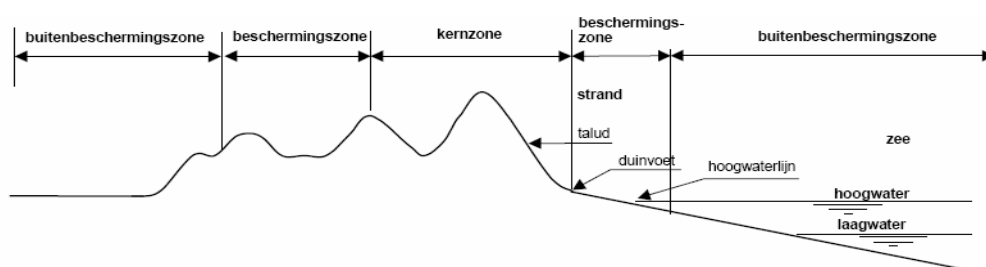
AFBEELDING 25.1 OVERZICHT LEGGERZONES ZEEWERING
