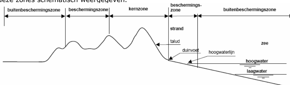
AFBEELDING 21.1 OVERZICHT LEGGERZONES ZEEWERING
