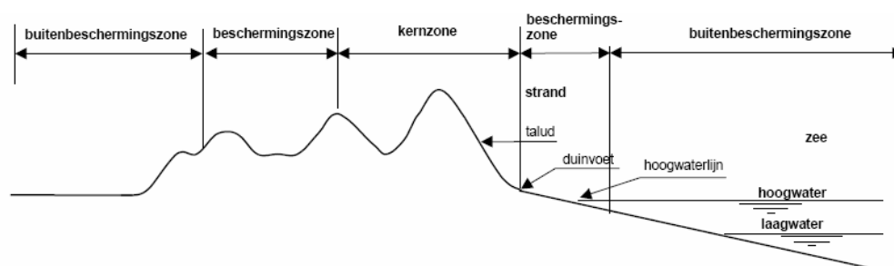
AFBEELDING 19.1 OVERZICHT LEGGERZONES ZEEKERING
