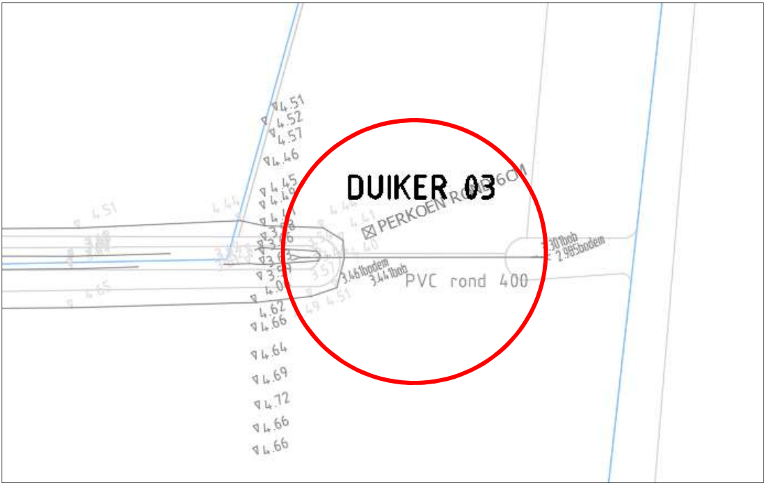
Aanpassingen in de Legger aan te leggen duiker
