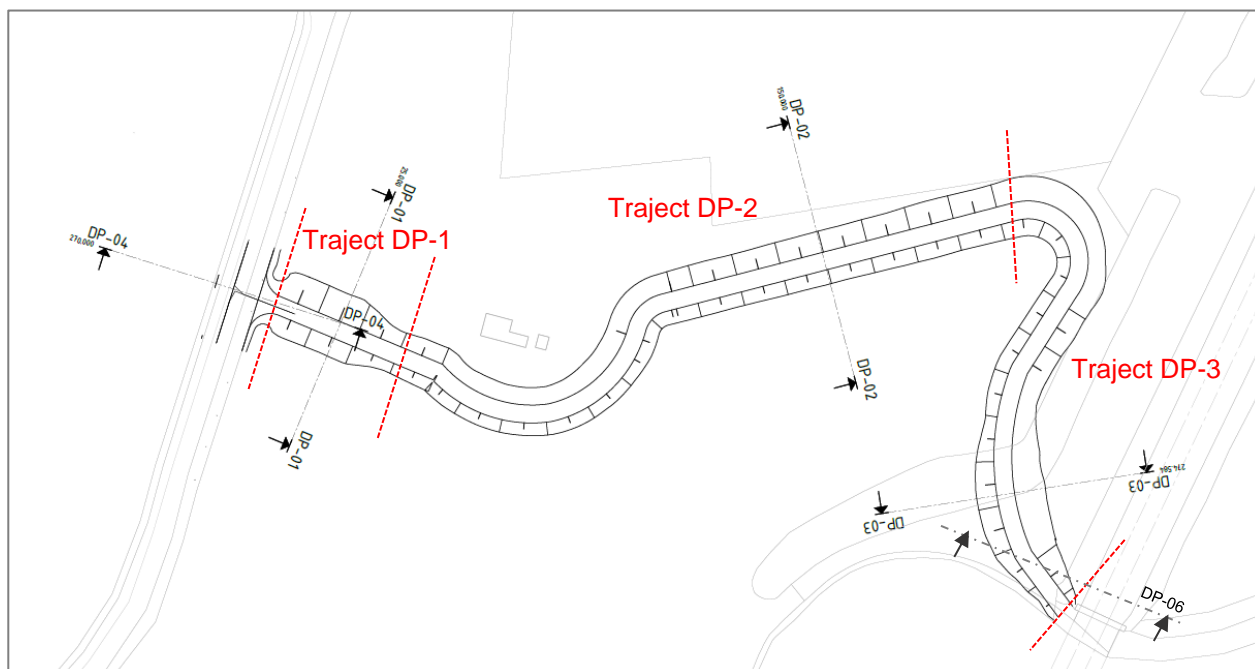
Figuur 2-2: Dwarsprofielen en trajectindeling nieuwe kade Drents Diep
