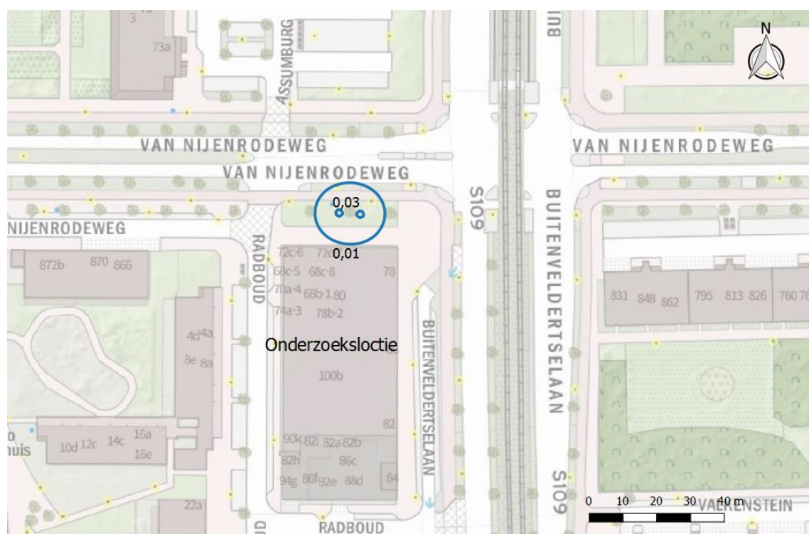
Figuur 4.1 Berekend hydrologisch invloedsgebied in WVP1, retourneren van 10 \text{ m}^3/\text{u} .
