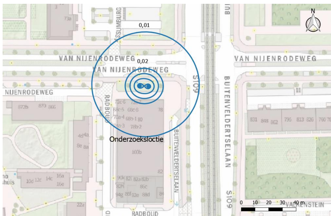
Figuur 4.2 Berekend hydrologisch invloedsgebied in WVP1, retourneren van 20 m³/u..
