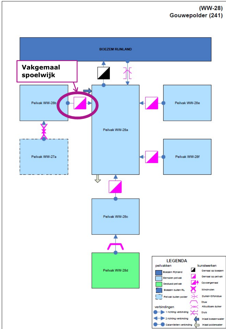
Afbeelding 2: Schematisatie Gouwepolder 1
