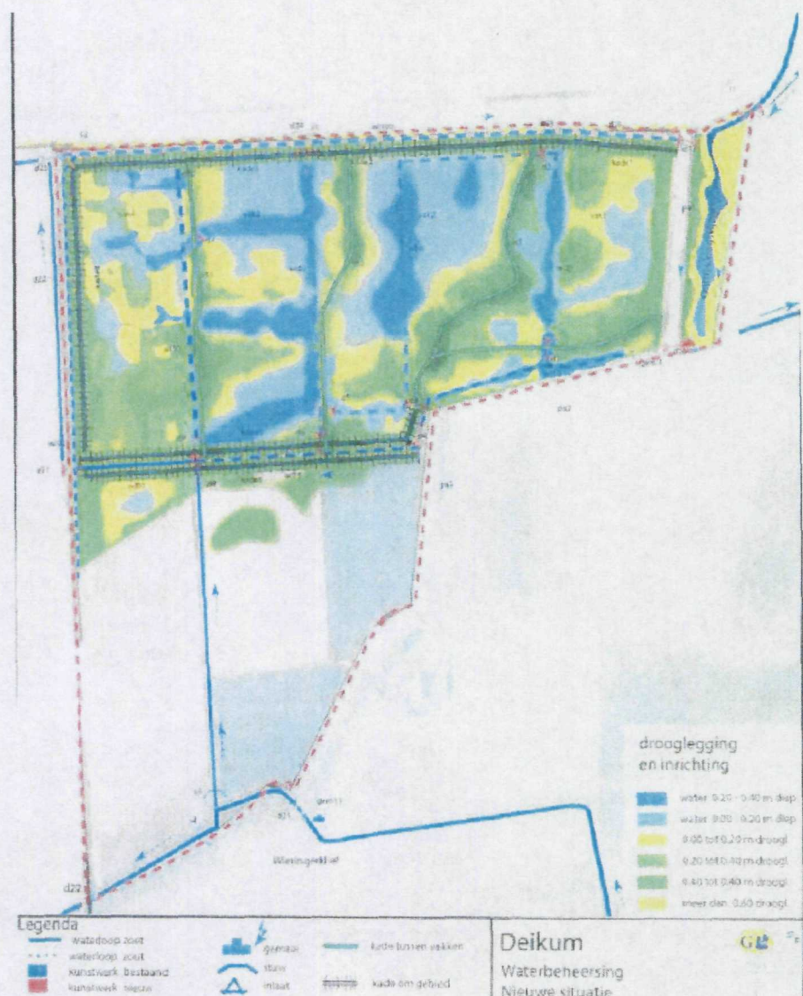
Figuur 1 Inrichtingstekening Deikum
