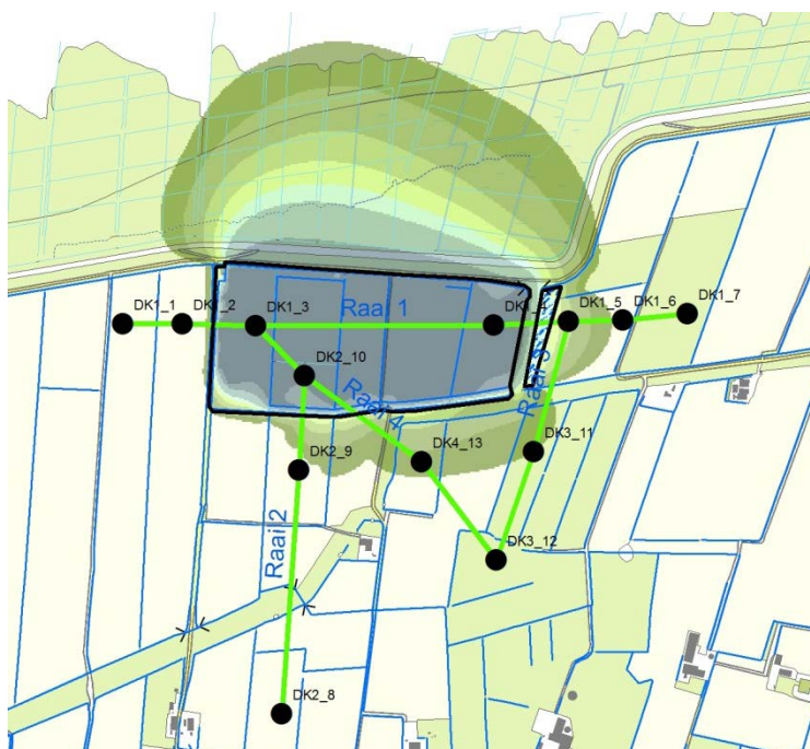
Afbeelding 6.1: voorstel peilbuismeetnet Deikum (zie ook figuurbijlage 30)
