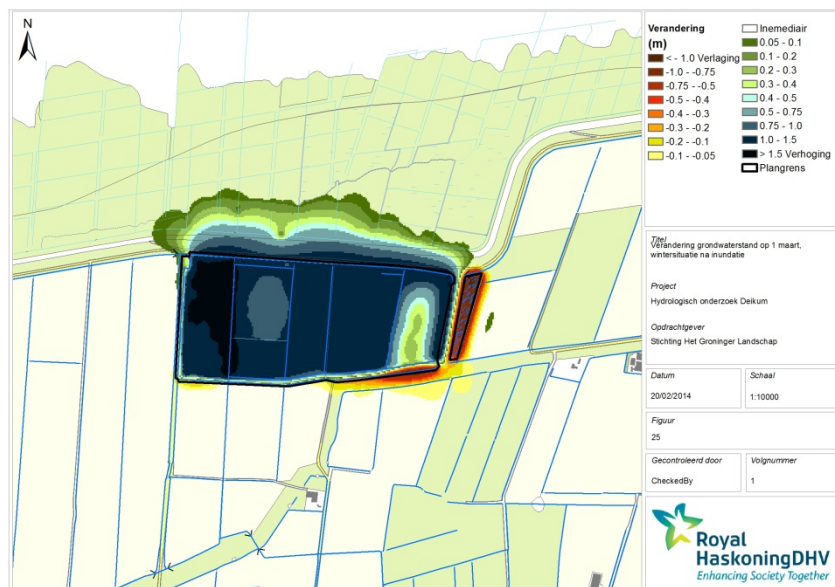
Afbeelding 3.16 Verandering grondwaterstand op 1 maart toekomstige wintersituatie na inundatie t.o.v. huidige wintersituatie (zie ook figuurbijlage 25).
