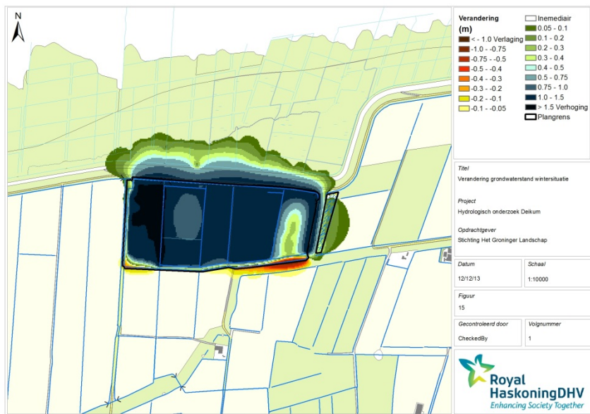
Afbeelding 3.6 Verandering grondwaterstand toekomstige wintersituatie t.o.v. huidige wintersituatie (zie ook figuurbijlage 15).
