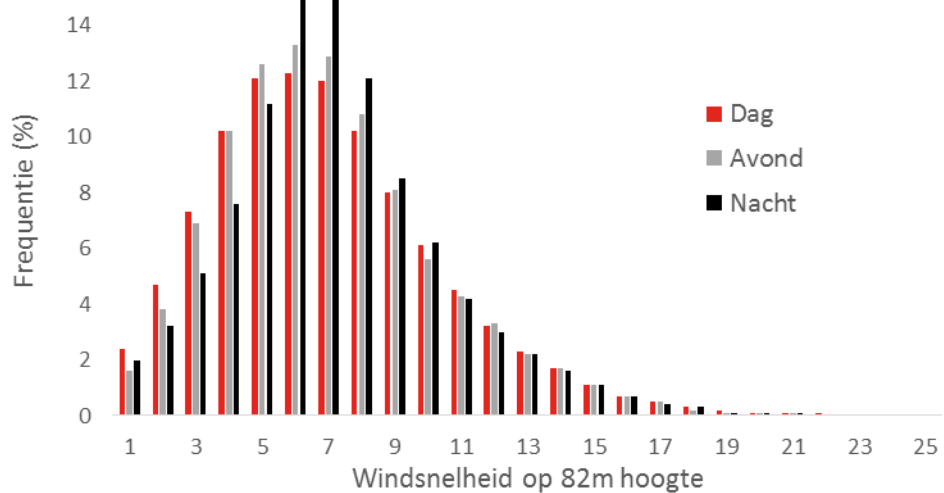
Figuur 3 Gegevens windsnelheid op 82m hoogte. Bron: KNMI 2018. Gemiddeld: 7,1 m/s.
