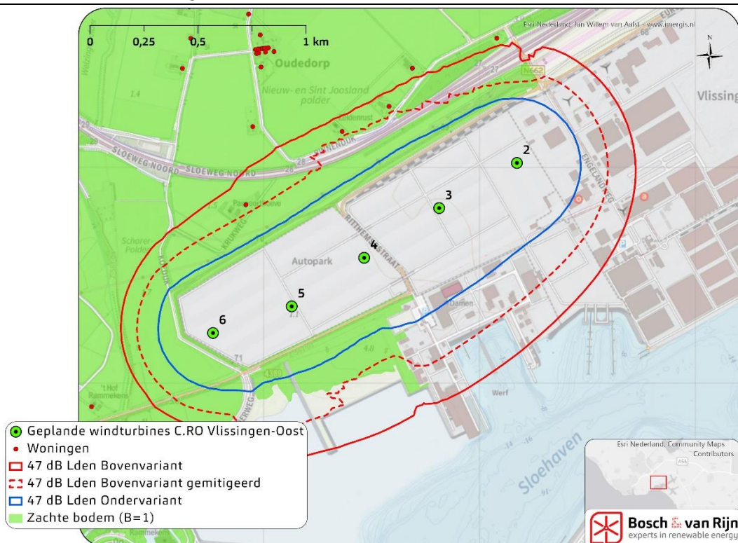
Figuur 6 Geluidscontour (47 dB L den ) van de bovenvariant, zowel met als zonder mitigatie in de vorm van reductiemaatregelen uit Tabel 5.
