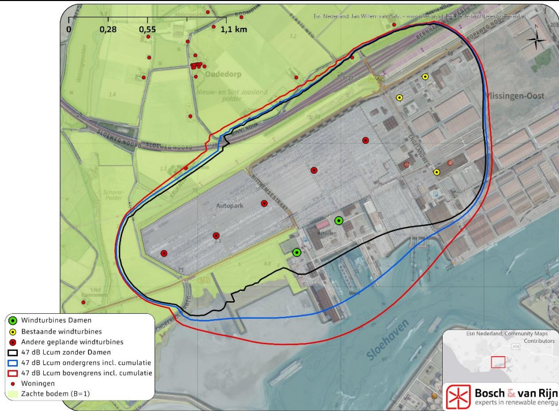
Figuur 7 Geluidscontouren (47 dB L den ) van bestaande en geplande windturbines (zwarte lijn), en de cumulatieve geluidscontour inclusief de ondergrens (blauw) en bovengrens (rood) voor de windturbines Damen Shipyards.
