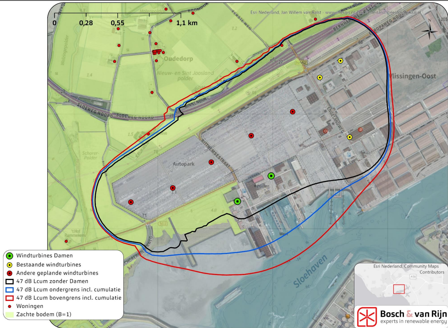
Figuur 7 Geluidscontouren (47 dB L_{den} ) van de bestaande en geplande windturbines (zwart) en daaraan toegevoegd de onder- en bovenvariant (blauw resp. rood).
