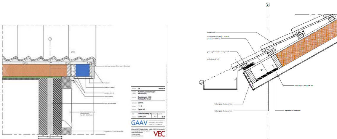
Figuur 3: Detail V5 permanente vleermuisverblijven (links) met aanvullende isolatie ( blauw vlak) Detail V6 permanente huismusverblijfplaatsen (rechts) Bron: Activiteitenplan Lieren complex 1903 (Loopplan, 2019) en email met aanvullingen van 2 september.
