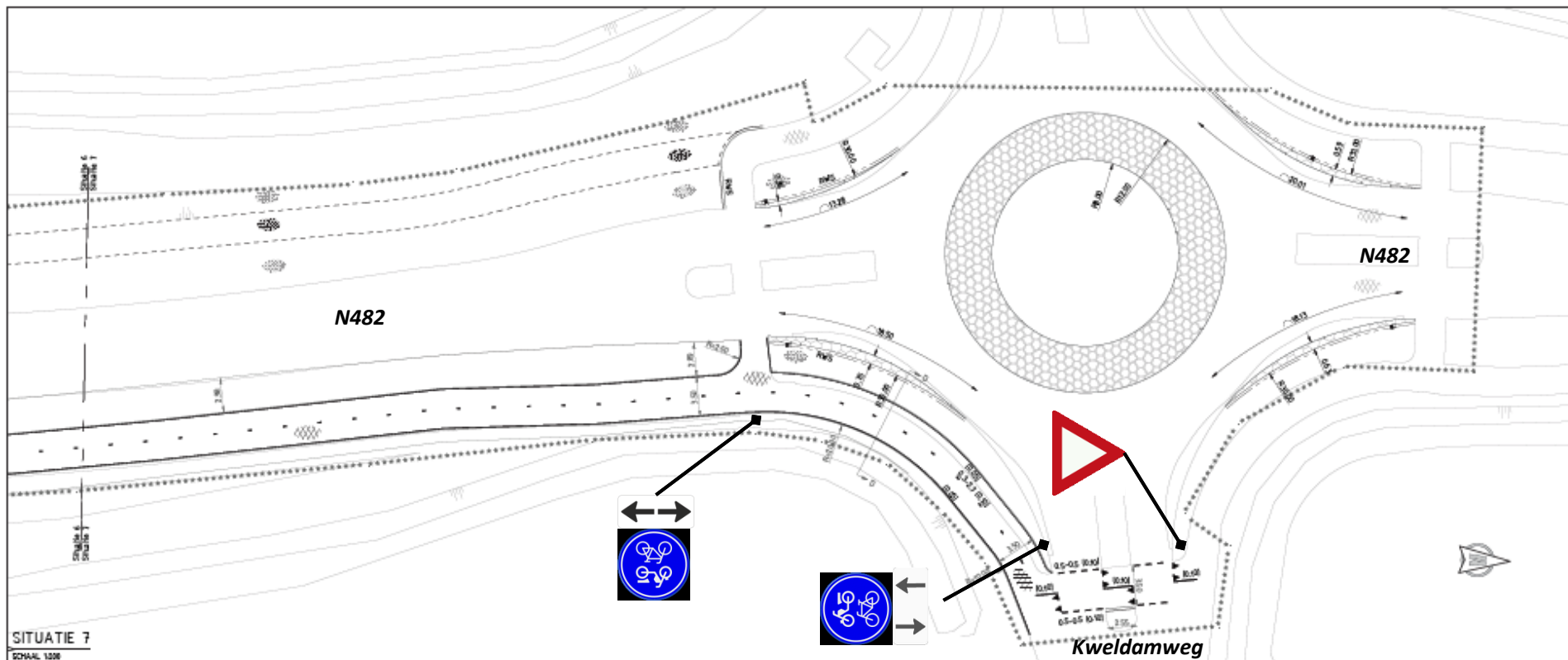
Tekening behorende bij Verkeersbesluit (brom)fietspad N482 PZH-VKB-N482-MW001 21 juni 2019
