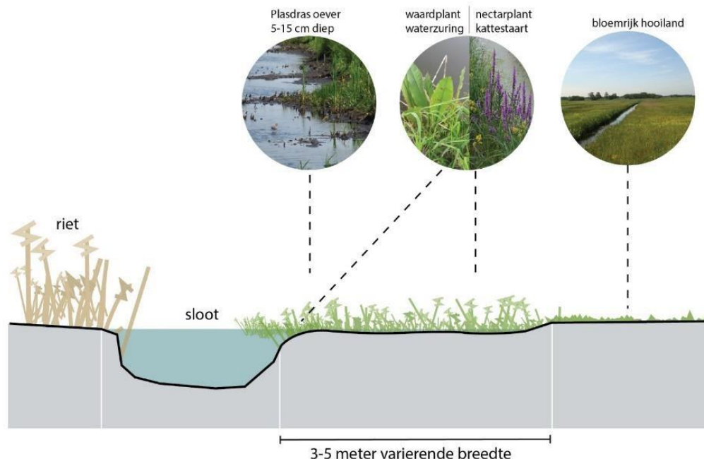
Figuur 1. Principeprofiel toekomstige oevers voor Grote vuurvliedder Omgeving Dwarsgracht.
