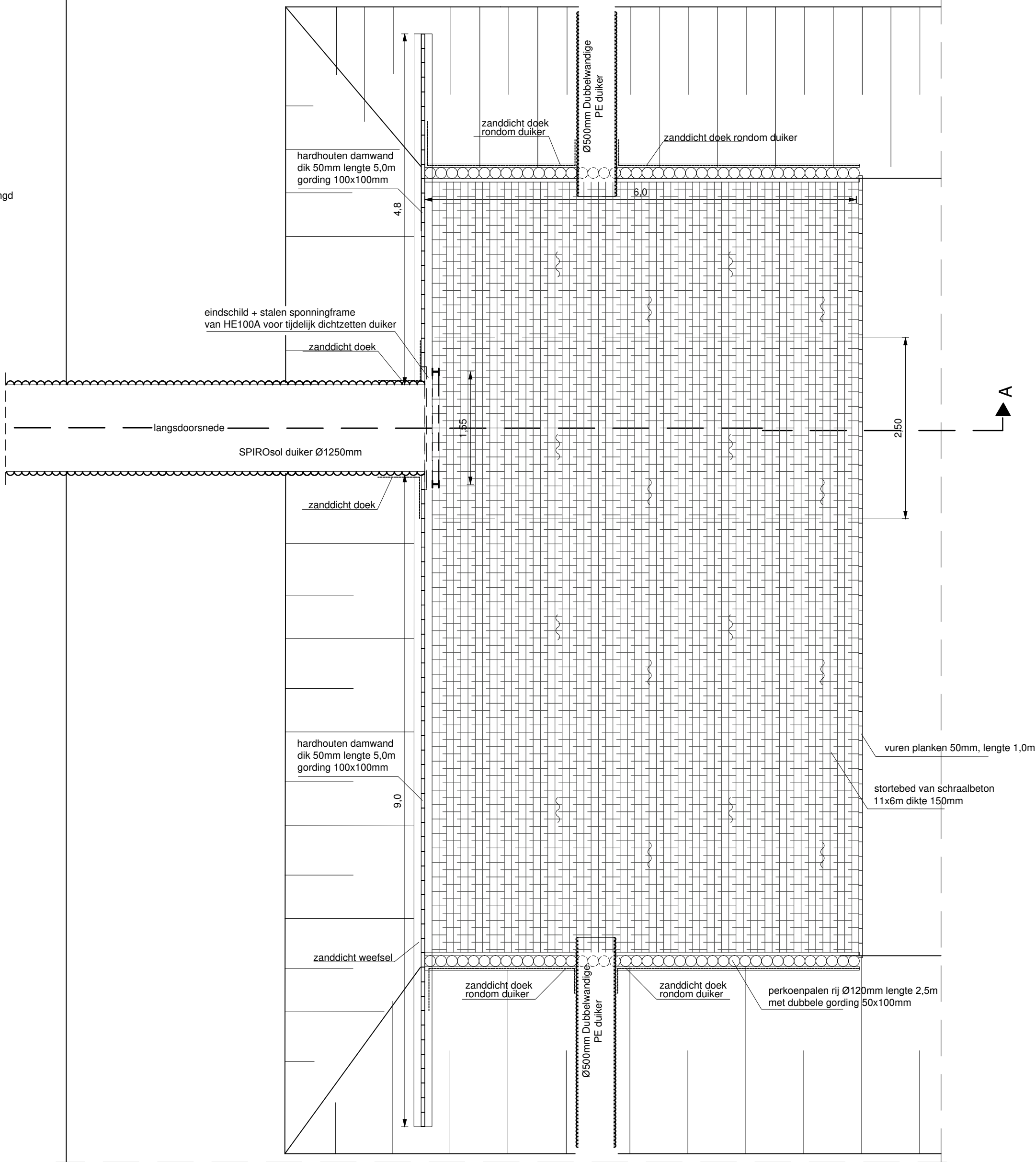
Diiker door Wierdijk Bovenaanzicht Schaal: 1:50
