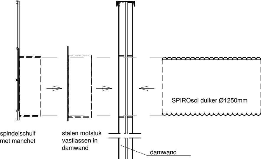
principe montage schuif/duiker detail Schaal: 1:n.v.t.
