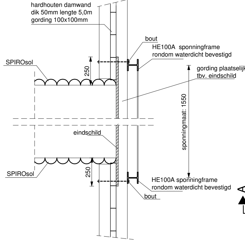
bevestiging stalen spinningsframe principe detail Schaal: 1:20
