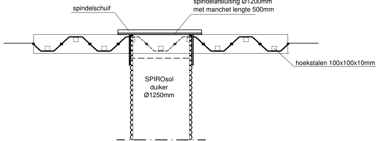
Diiker door Wierdijk Bovenaanzicht Schaal: 1:50
