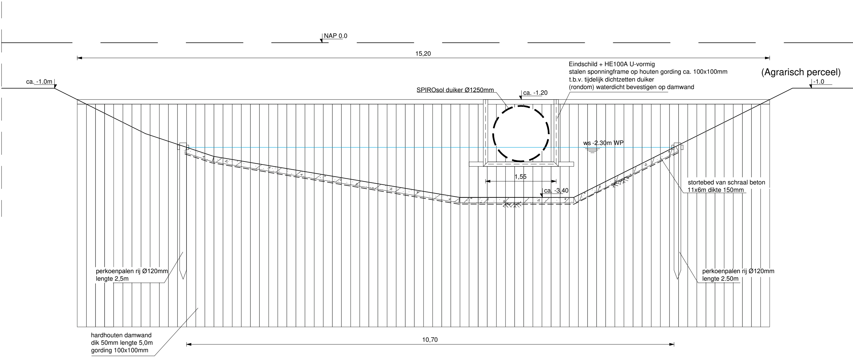
Diiker door Wierdijk Vooraanzicht Schaal: 1:50
