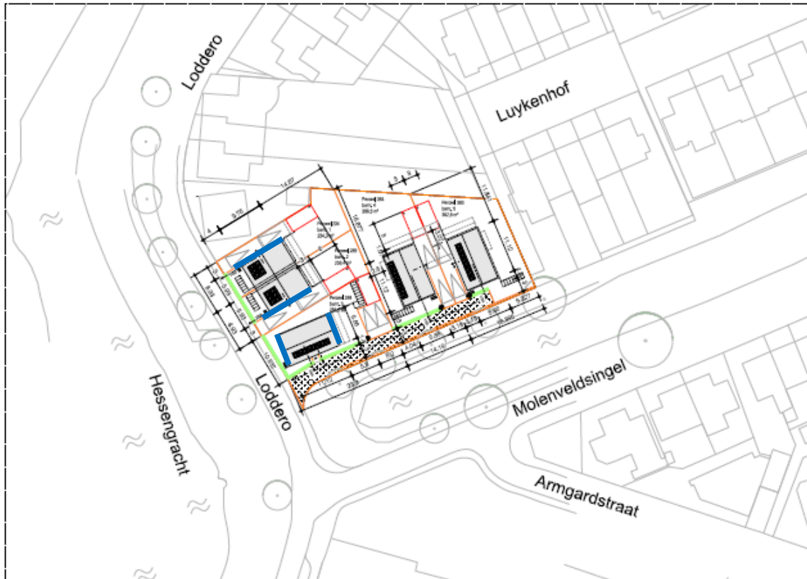
Figuur 3. Locaties permanente voorzieningen in de nieuwbouw (blauwe lijnen). Elke lijn staat voor twee inbouwvloermuiskasten van het type Schwegler 1FF.
