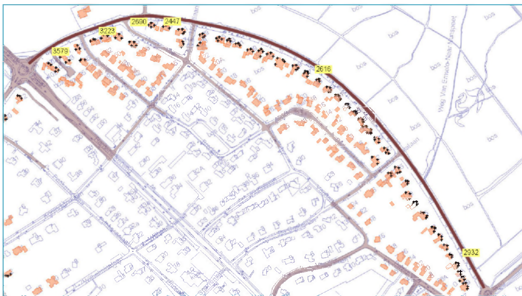
Figuur 4 Verkeersintensiteiten per etmaal Jacob Catslaan 2030
