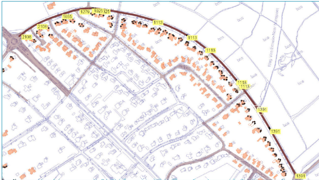
Figuur 3 Verkeersintensiteiten per etmaal Jacob Catslaan 2015
