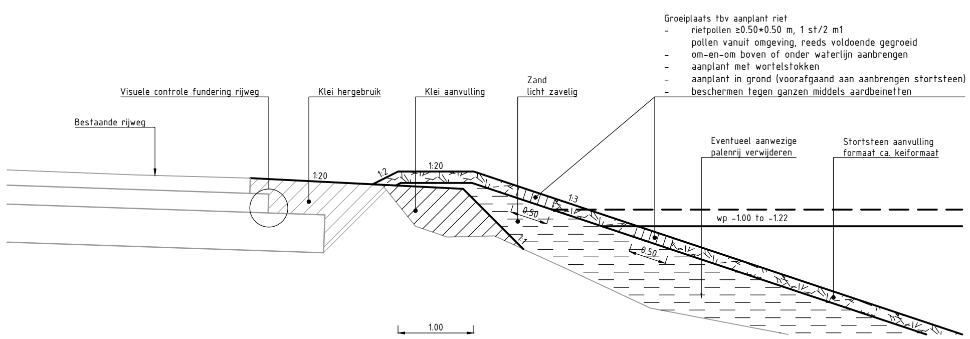
Principedwarsprofiel SCHAAL 1 : 50
