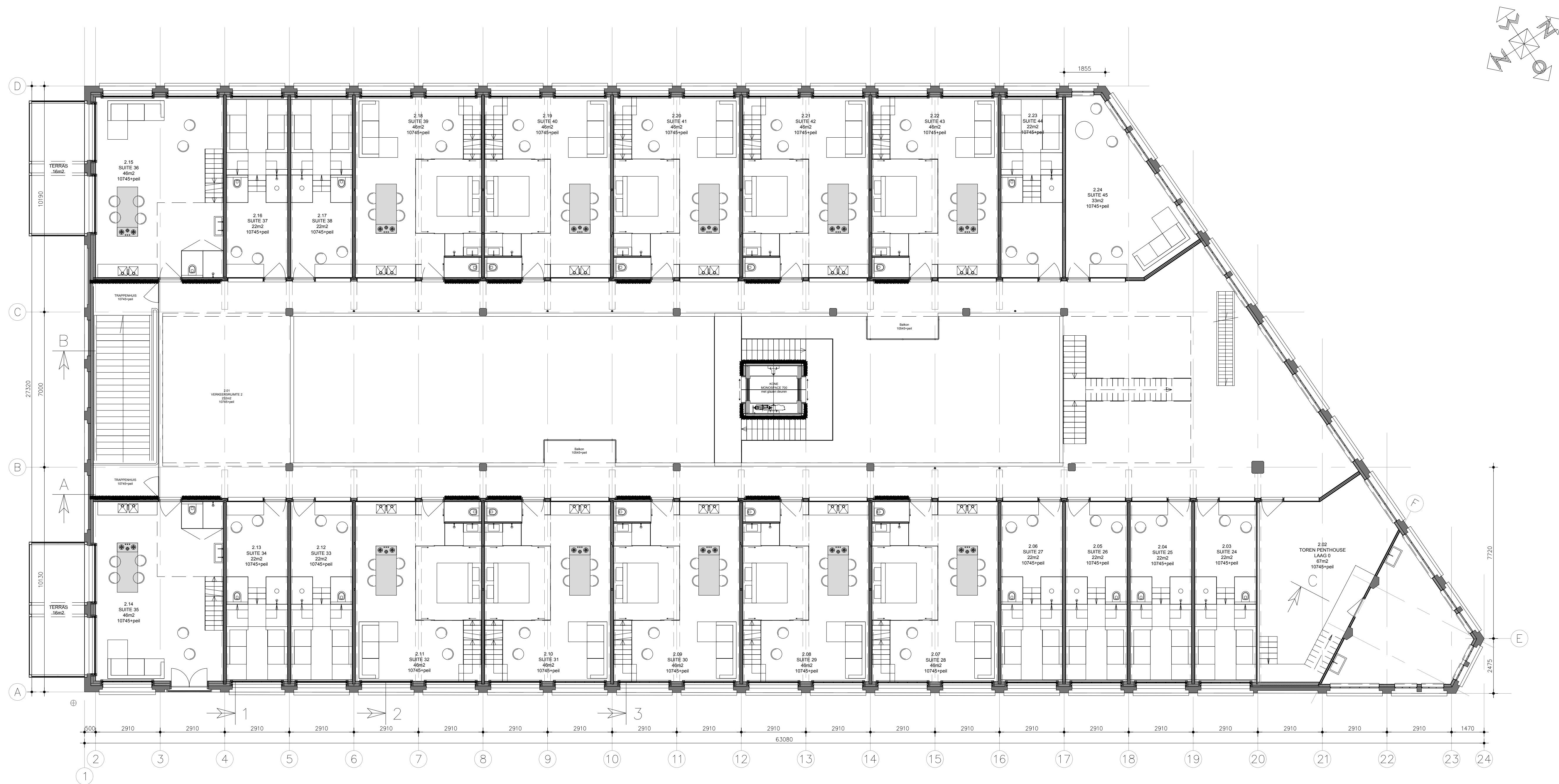
Tweede verdieping
