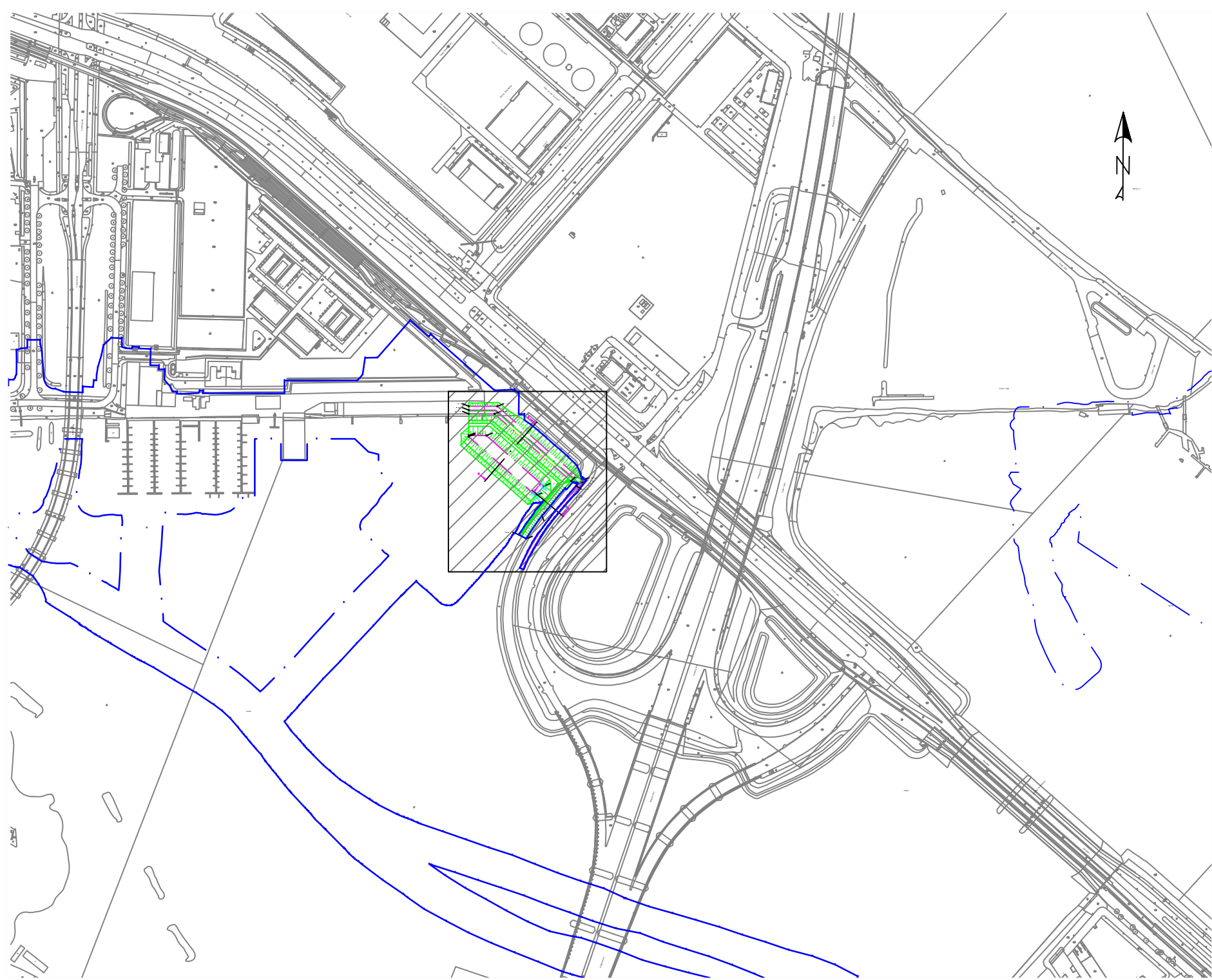
Situatie na de ontgraving t.b.v. aanleggen van de bekleding
