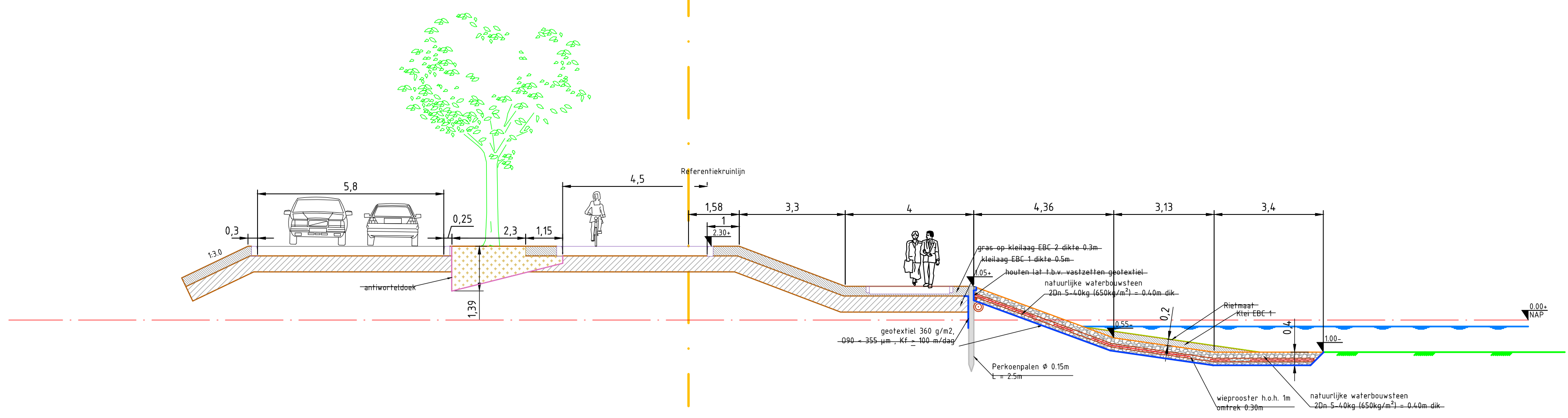
Dwarsprofiel B SCHAAL 1 : 1000
