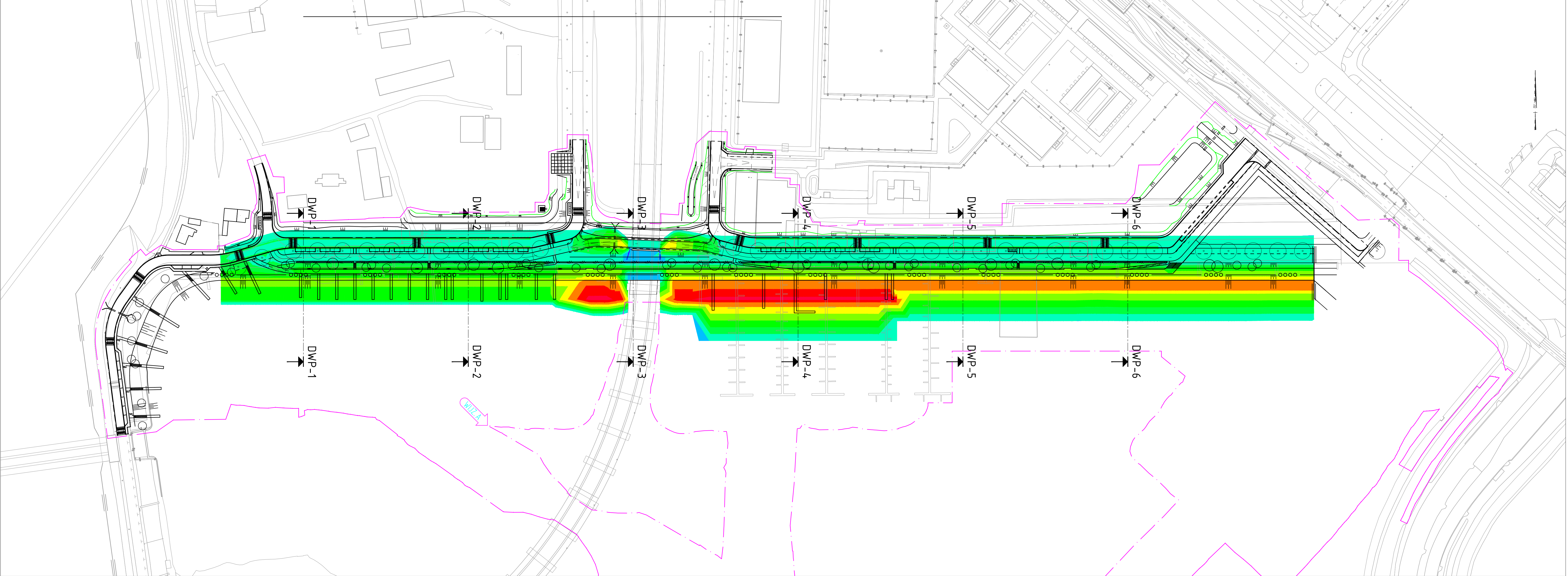
Overzicht grondwerk SCHAAL 1:1500
