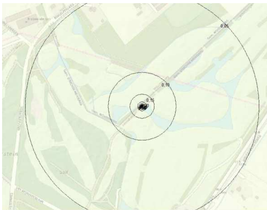
Fig. 4.2: Berekende verlaging [m], Scenario B, 3 de watervoerend pakket
