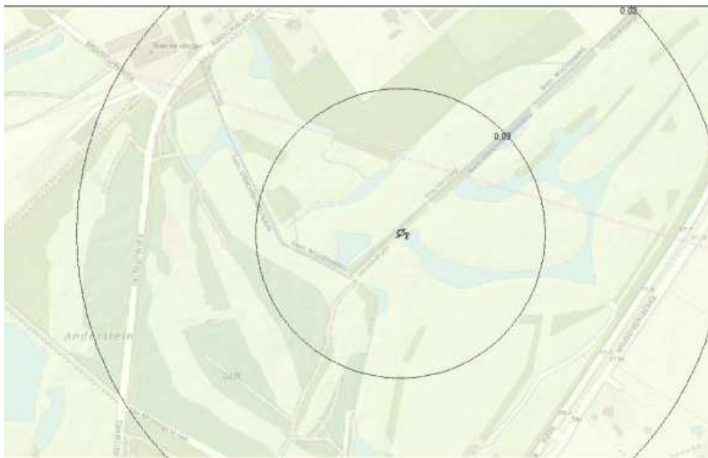
Fig. 4.1: berekende verlaging [m], Scenario A, 1 ste watervoerend pakket (freatisch)
