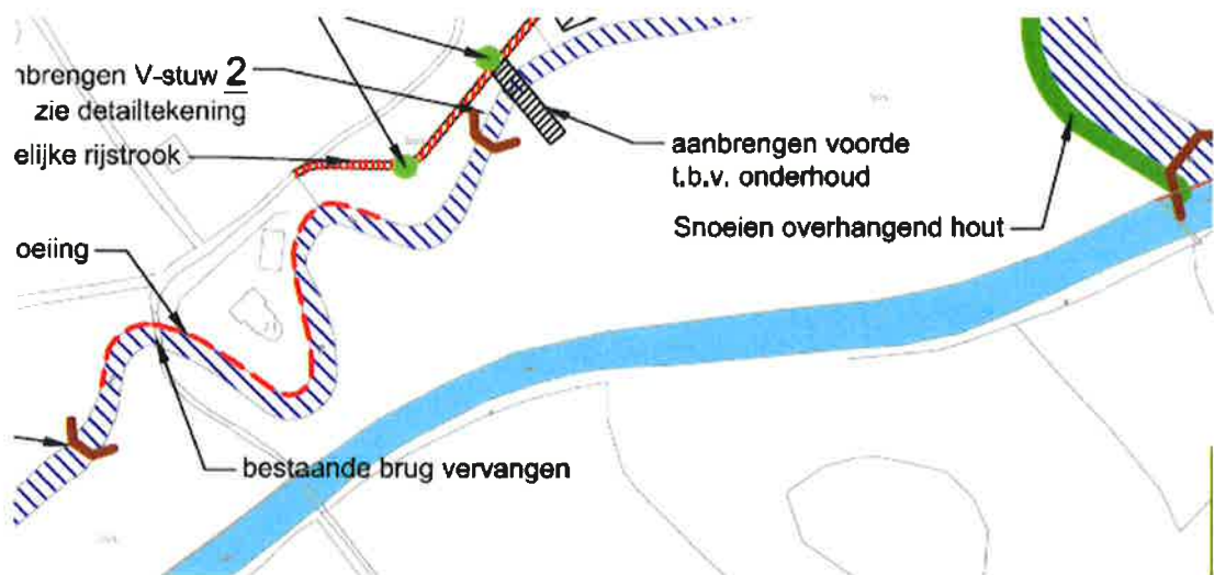
Situatietekening voorde
