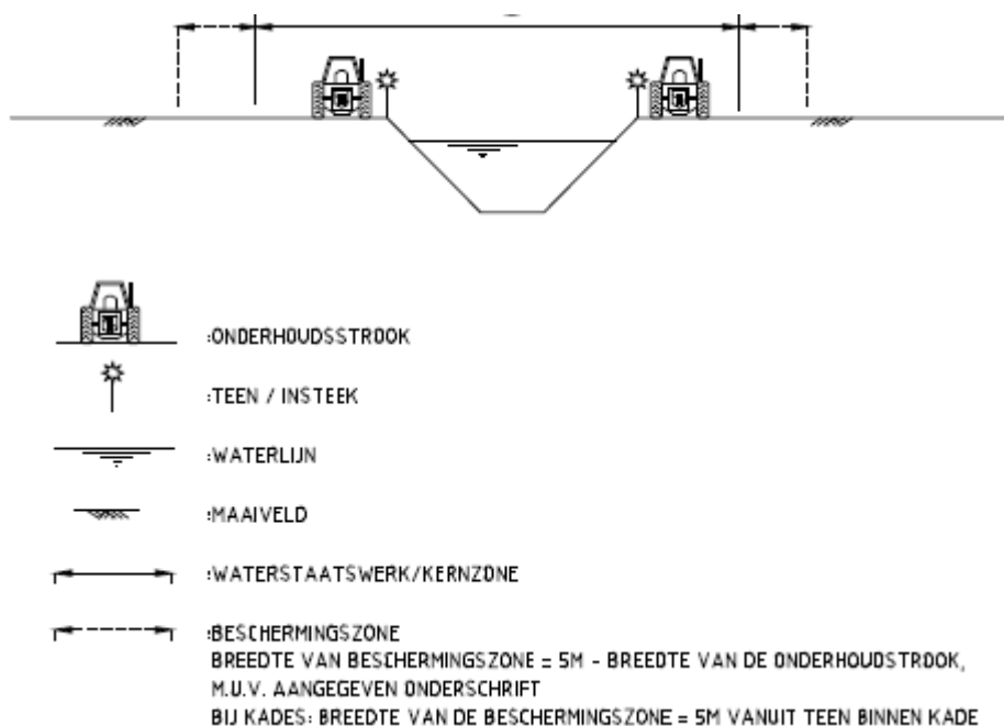
figuur 2.1 schematische weergave van de kernzone en beschermingszone van een watergang
