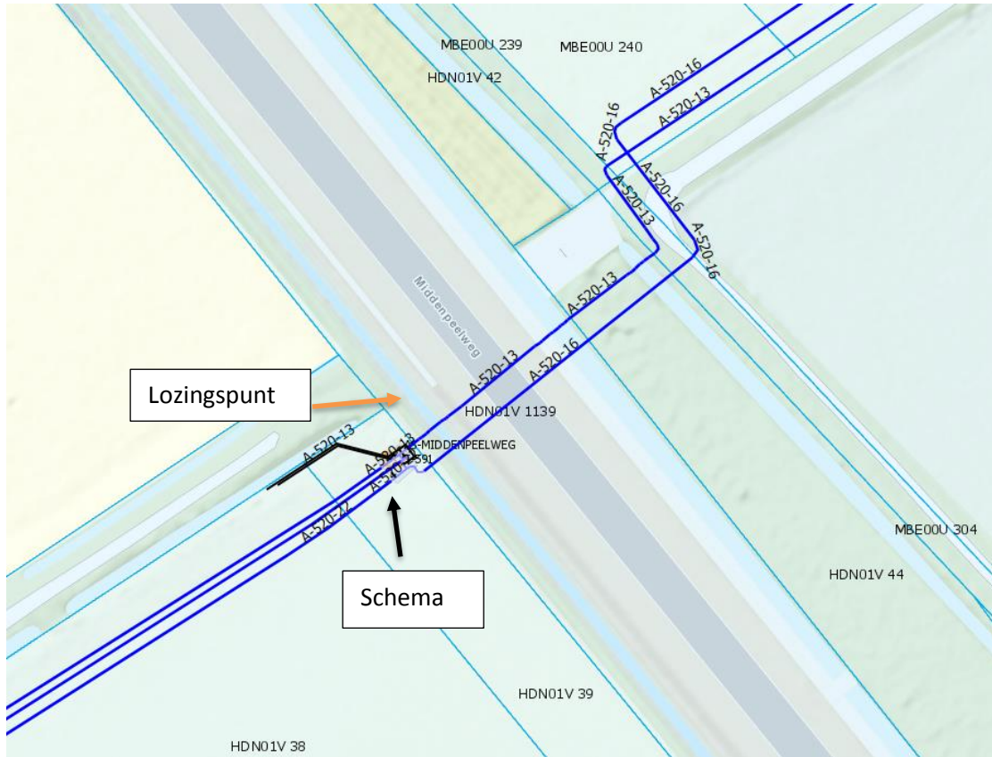
Te plaatsen bronnering bij schema S-591 nabij Oude Heldenseweg/Midden Peelweg in Helden.
