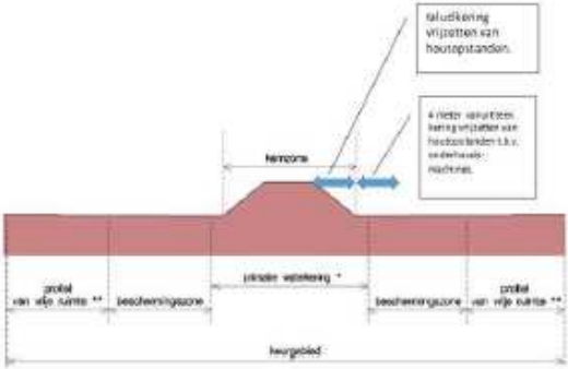
Dwarsprofiel waterkering
