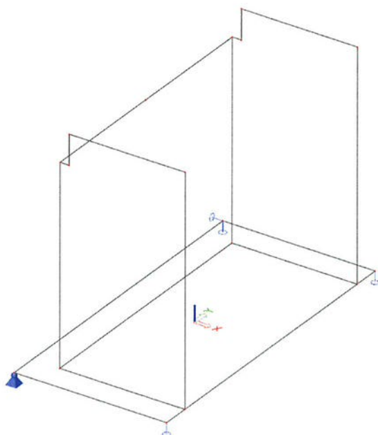
Figuur 11: Assenstelsel rekenmodel.
