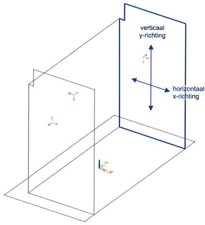
Figuur 17: Langs- en dwarsrichting vleugelwanden.
