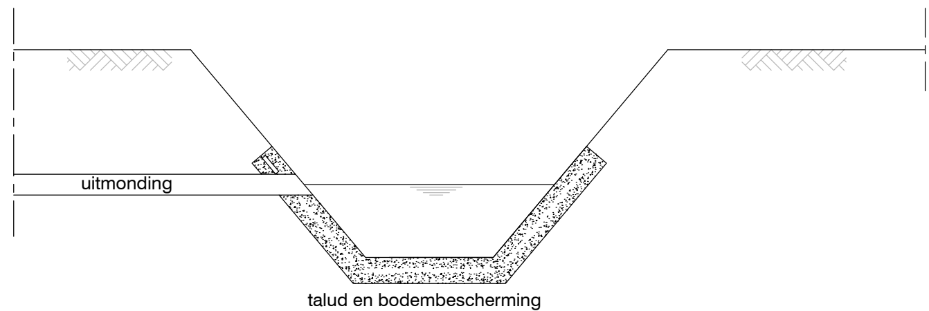
Dwarsdoorsnede A-A
