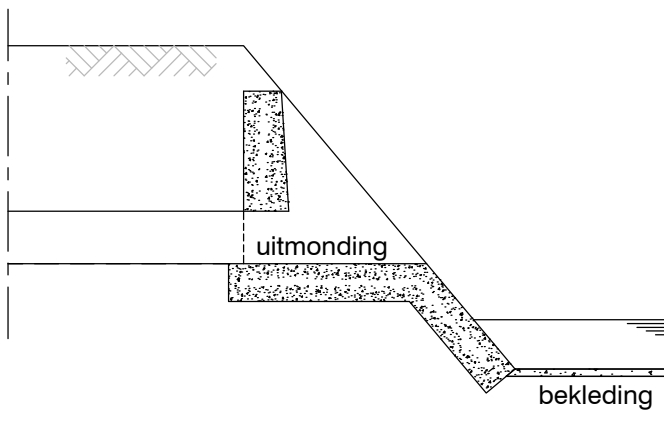
Dwarsdoorsnede A-A
