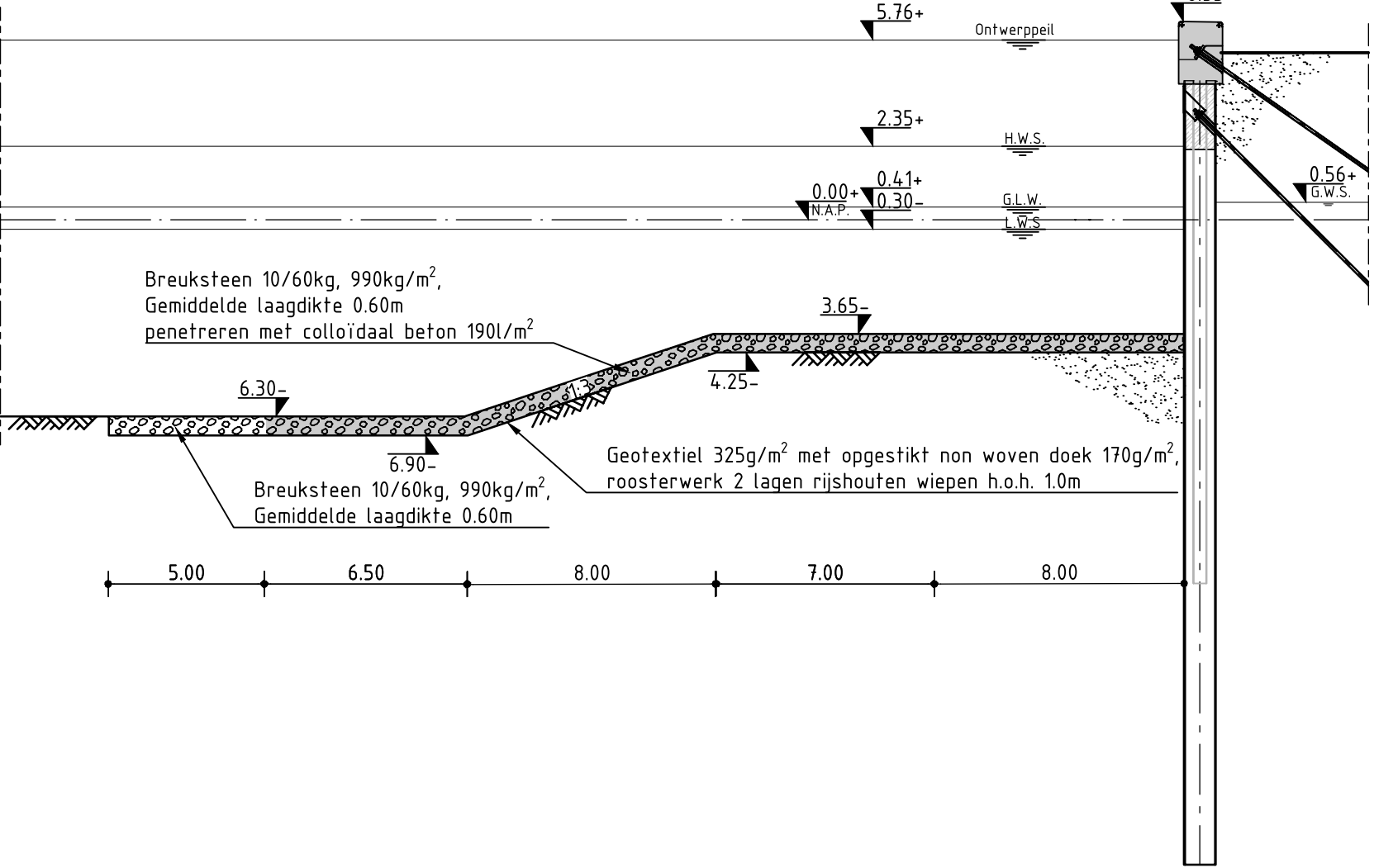
DOORSNEDE 02 - AANSLUITING OP BESTAANDE SLUIS SCHAAL 1:200
