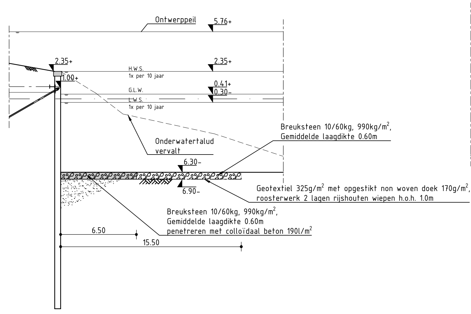
DOORSNEDE 01 - WESTZIJDE SCHAAL 1:200
