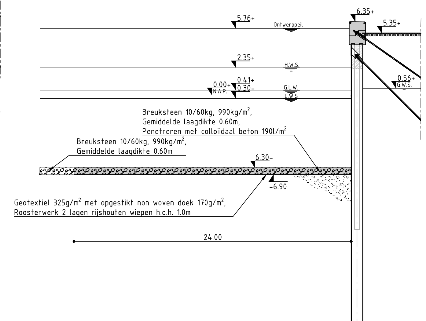
DOORSNEDE 04 - OOSTZIJDE SCHAAL 1:200
