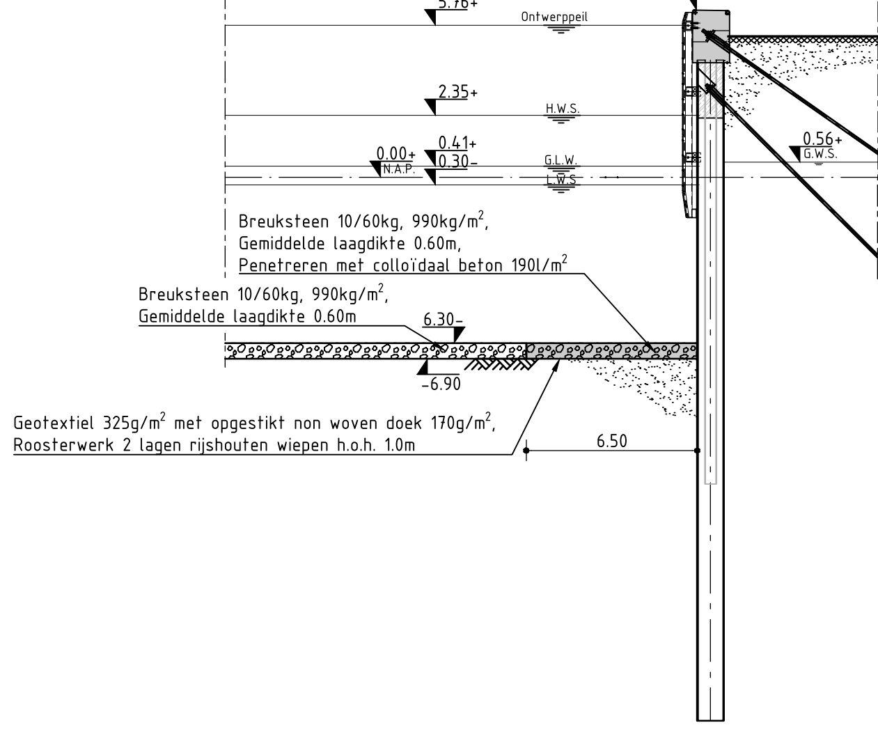
DOORSNEDE 03 - ZUIDZIJDE SCHAAL 1:200
