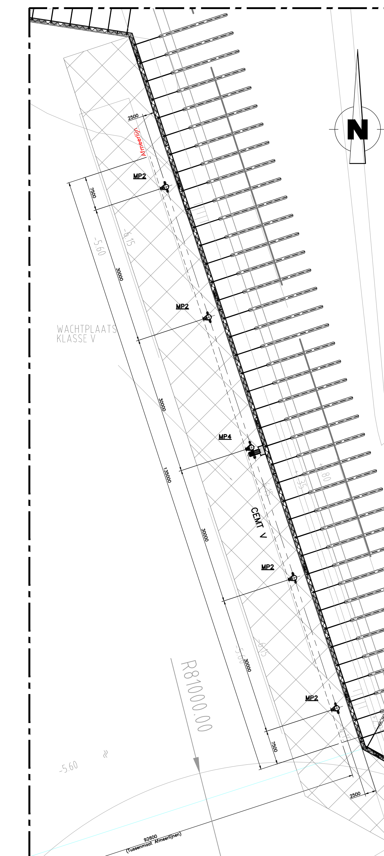
SITUATIE SCHAAL 1:500
