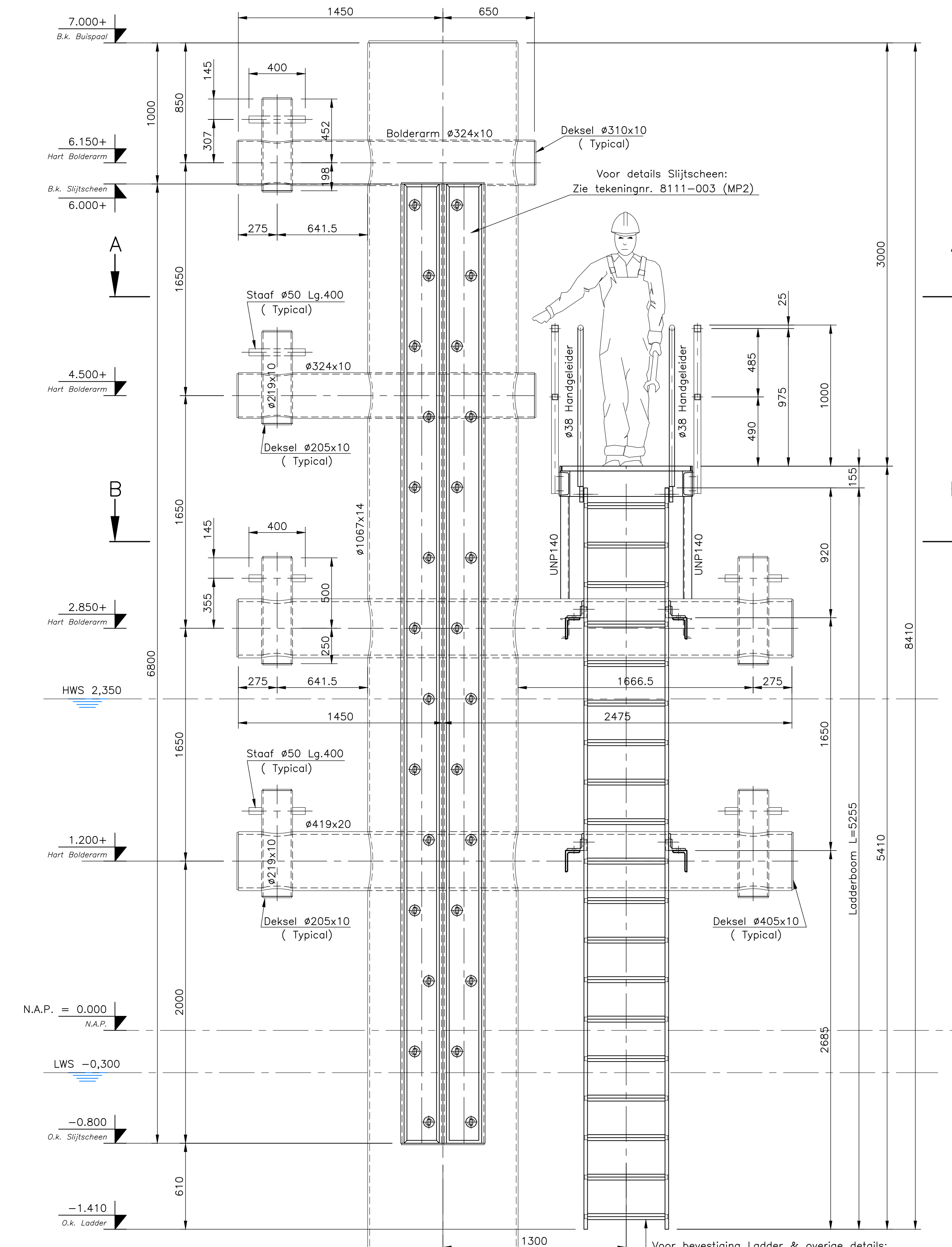
VOORAANZICHT MP4 PAAL & LADDER SCHAAL 1:20
