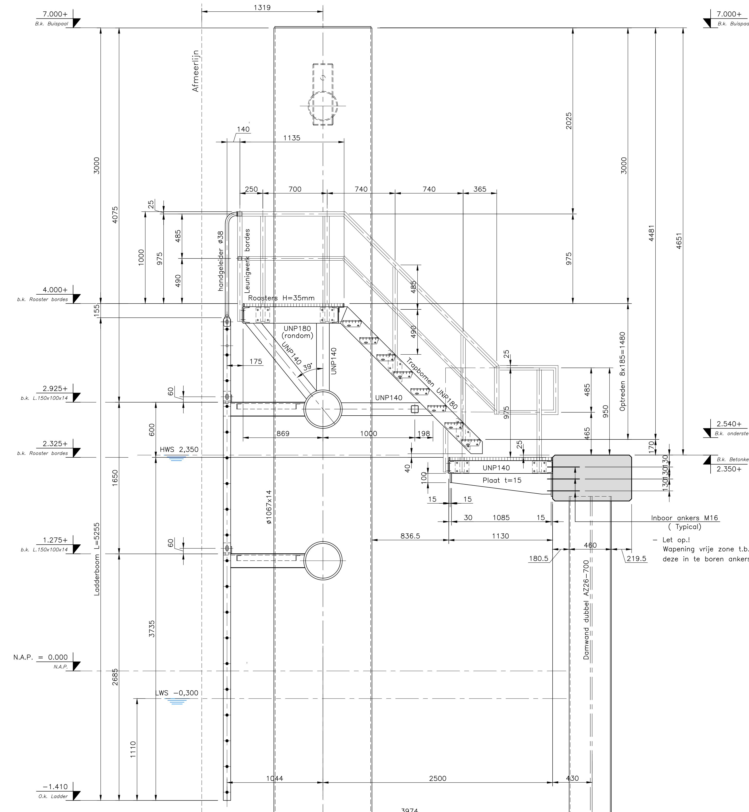
ZIJ-AANZICHT D-D MP4 PAAL, LADDERS & BORDESSEN SCHAAL 1:20
