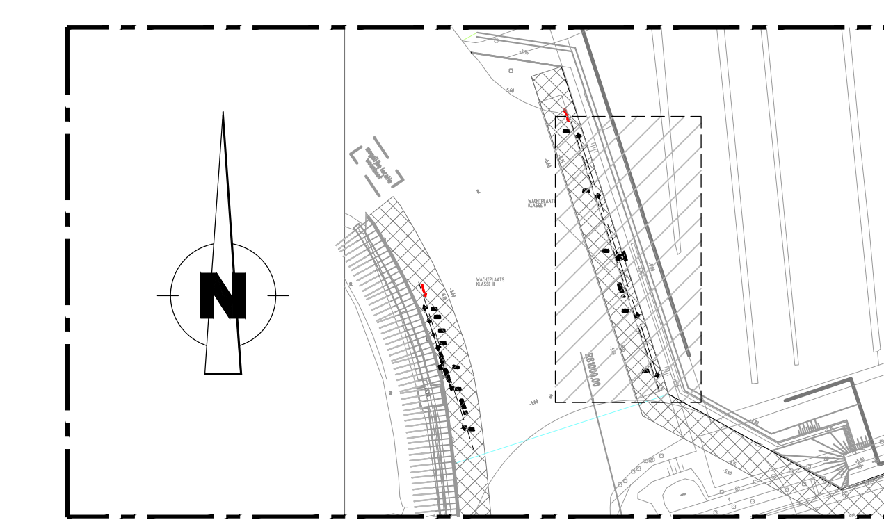
SITUATIE SCHAAL 1:2500
