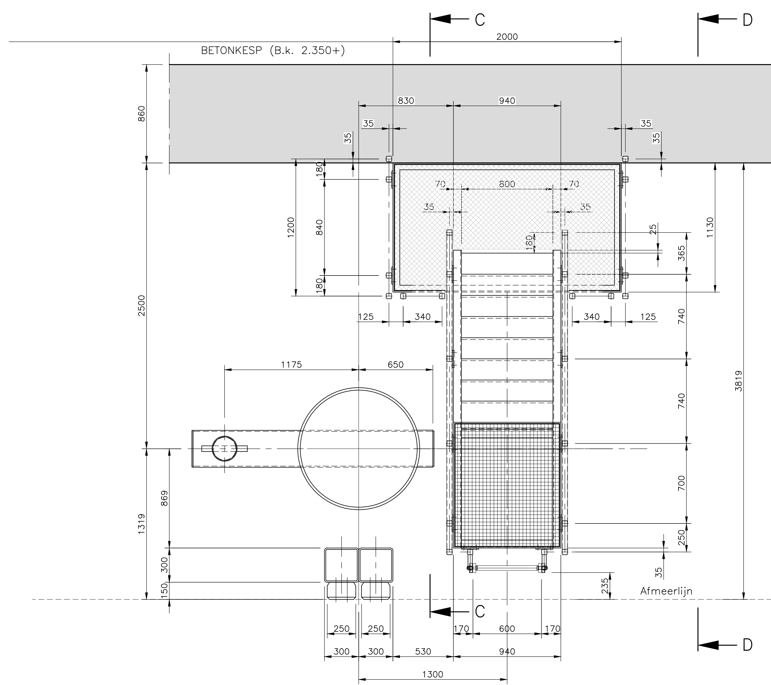
BOVENAANZICHT A-A Bordes +4000 SCHAAL 1:20
