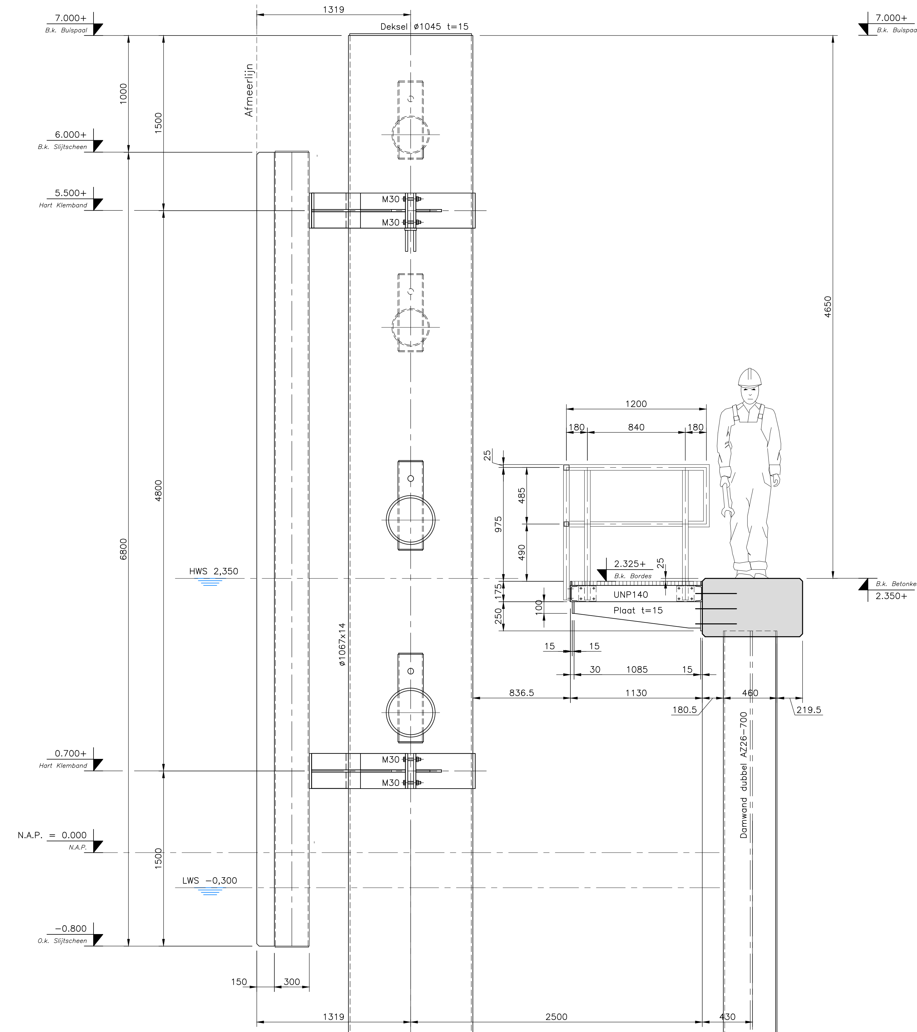
DOORSNEDE C-C MP4 PAAL & BORDES SCHAAL 1:20
