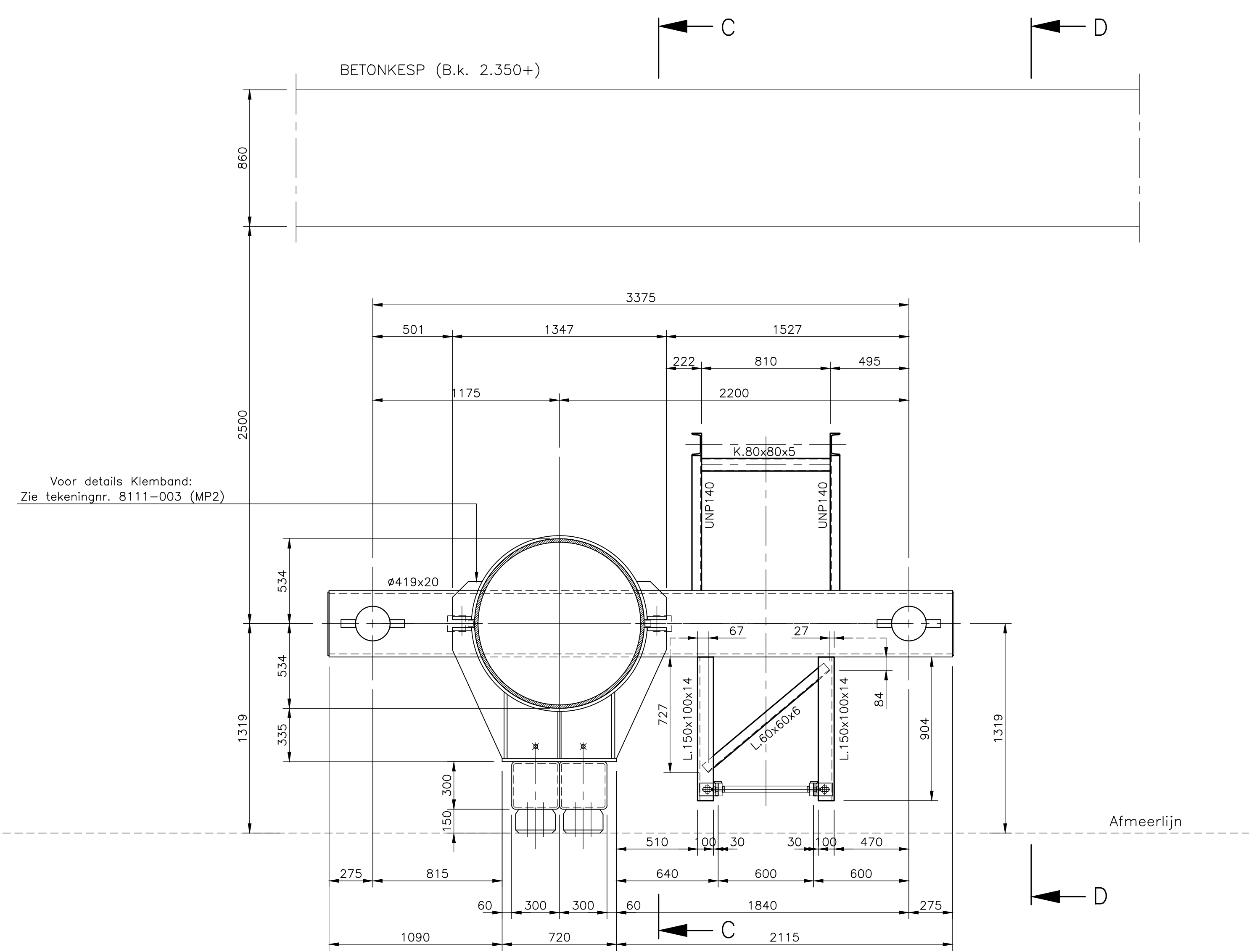
HORIZONTALE DOORSNEDE B-B (Ladderbevestiging) SCHAAL 1:20
