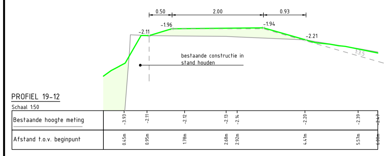
OVERZICHT C schaal 1:200
