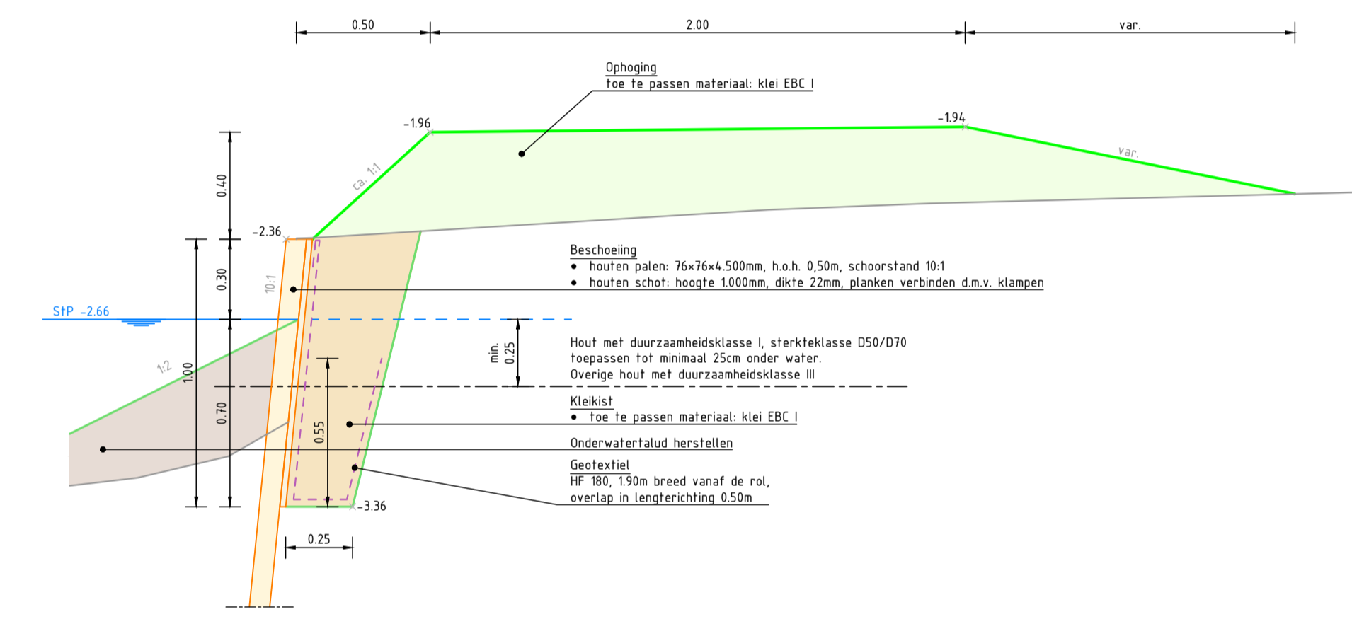
Principedetail Schaal 1:20
