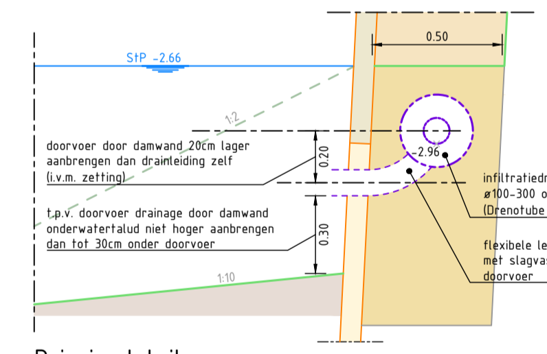
Principedetail Doorvoer infiltratiedrain door keerwand schaal 1:20
