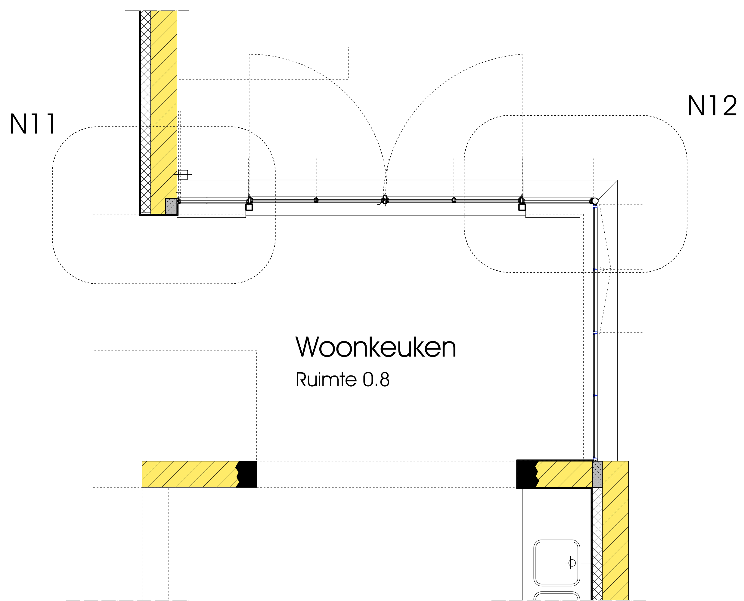
PLATTEGROND P+1500
