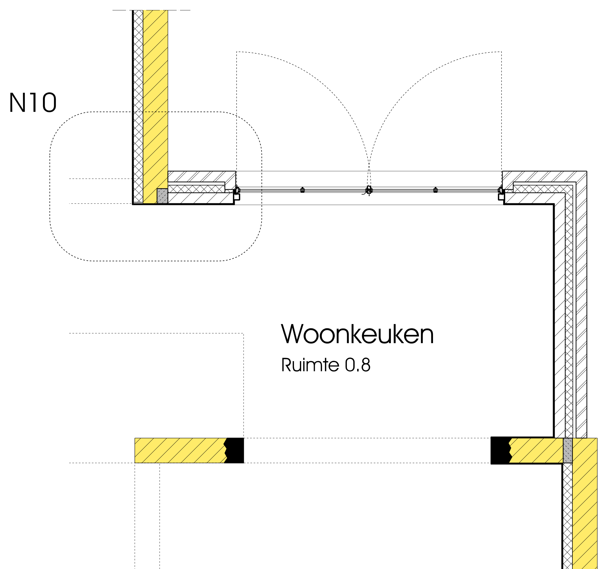
PLATTEGROND P+1000
