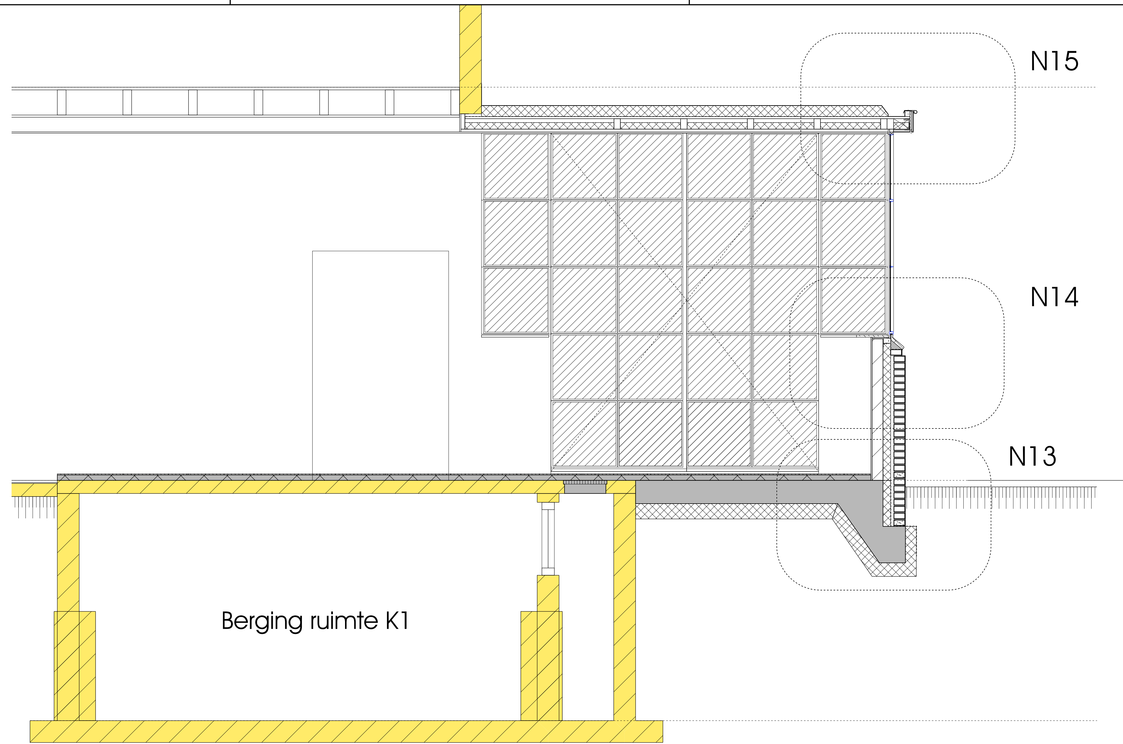
DOORSNEDE C-C
