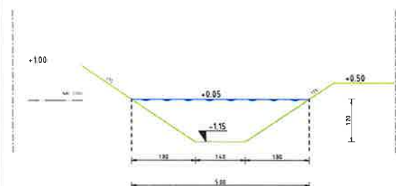
Principeprofiel A-A: watergang Haarpad 1:50
