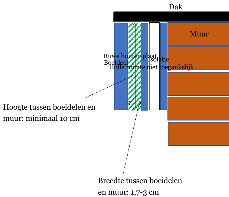
Figuur 1. Schematische weergave afmetingen permanente voorzieningen voor vleermuizen (groen gearceerd) achter nieuw te plaatsen boeidelen: breedte 1,7-3 cm en hoogte minimaal 10 cm.
