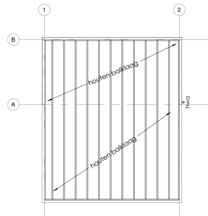
KAPPLAN
