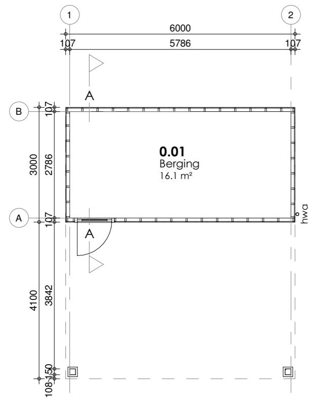
BEGANE GROND
