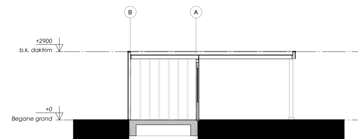
DOORSNEDE A-A
