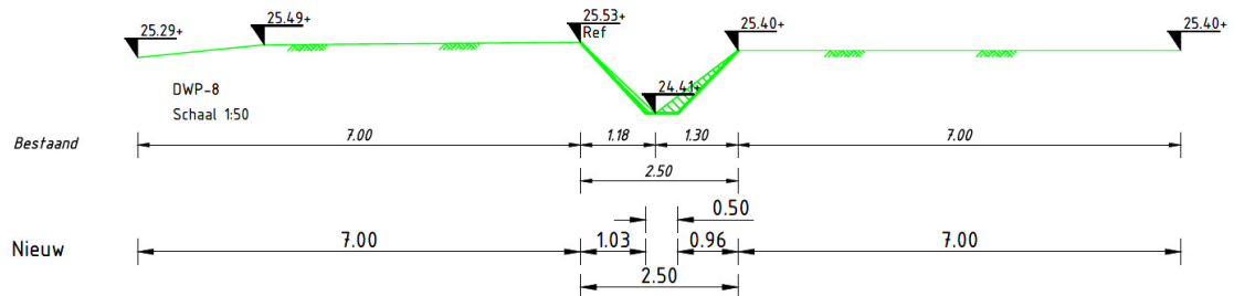
Figuur 2-6: Ontwerpprofiel Schelkensbeek secundair
