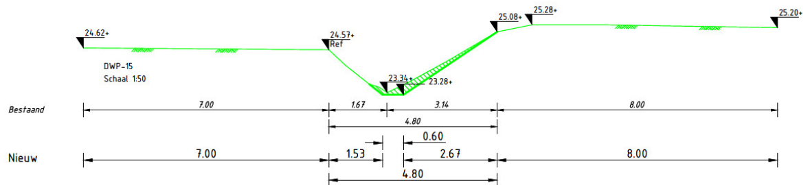
Figuur 2-5: Ontwerpprofiel Schelkensbeek - A73
