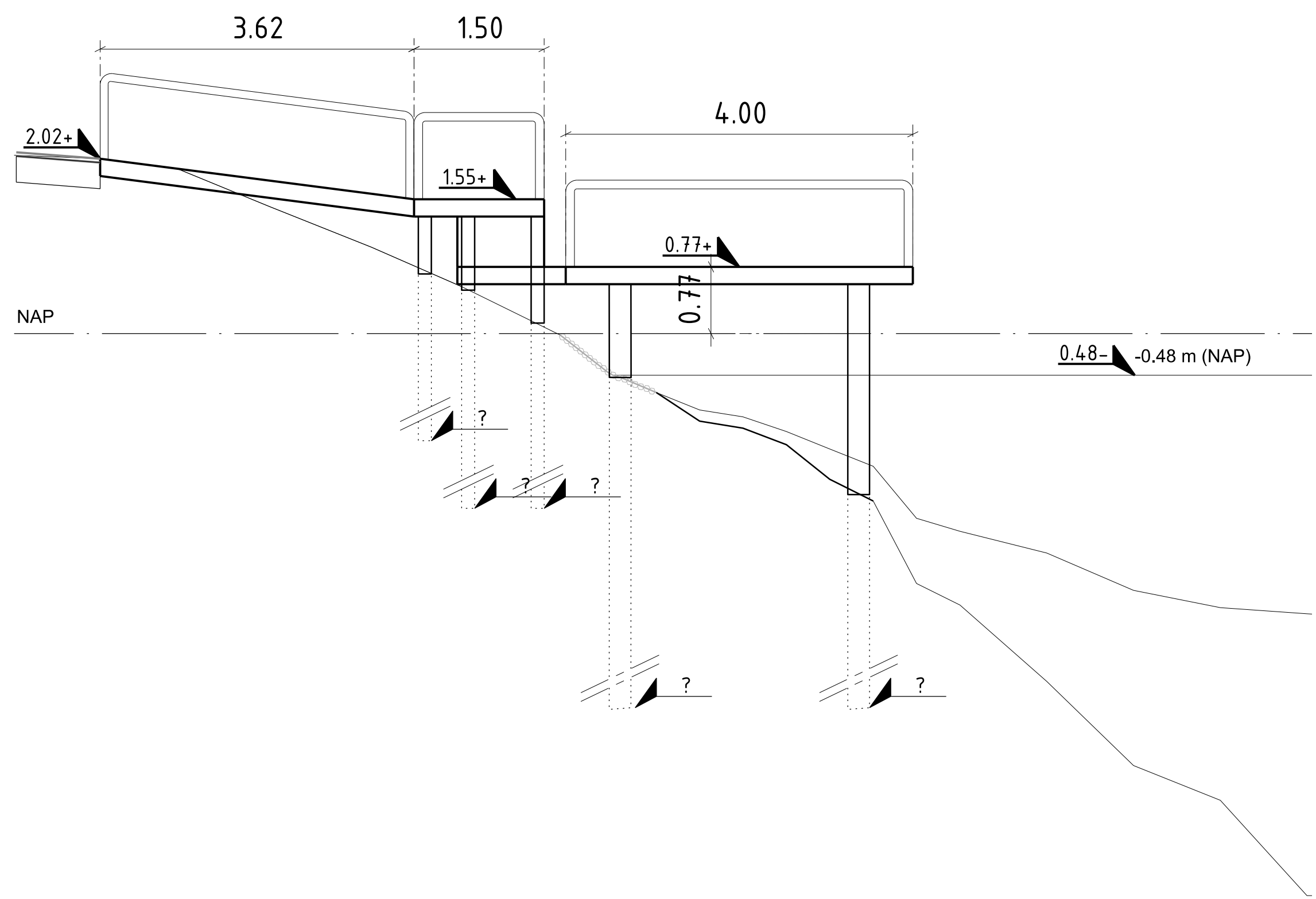
Zijaanzicht B - B vlonder nieuw SCHAAL 1 : 50
