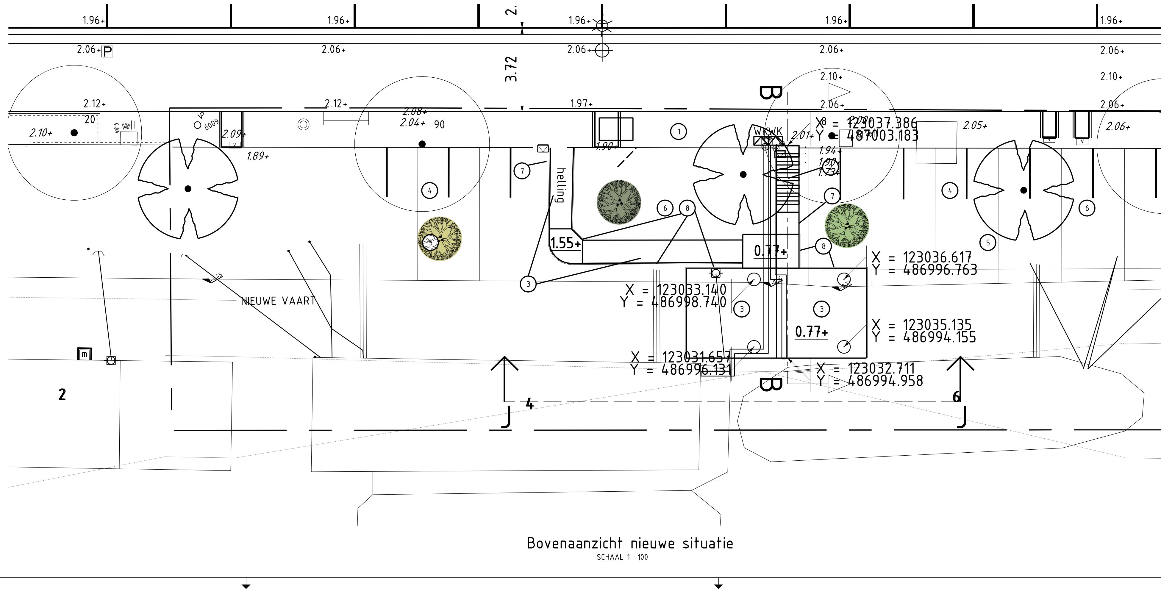
Bovenaanzicht kabels en leidingen en nieuwe situatie SCHAAL 1 : 100
