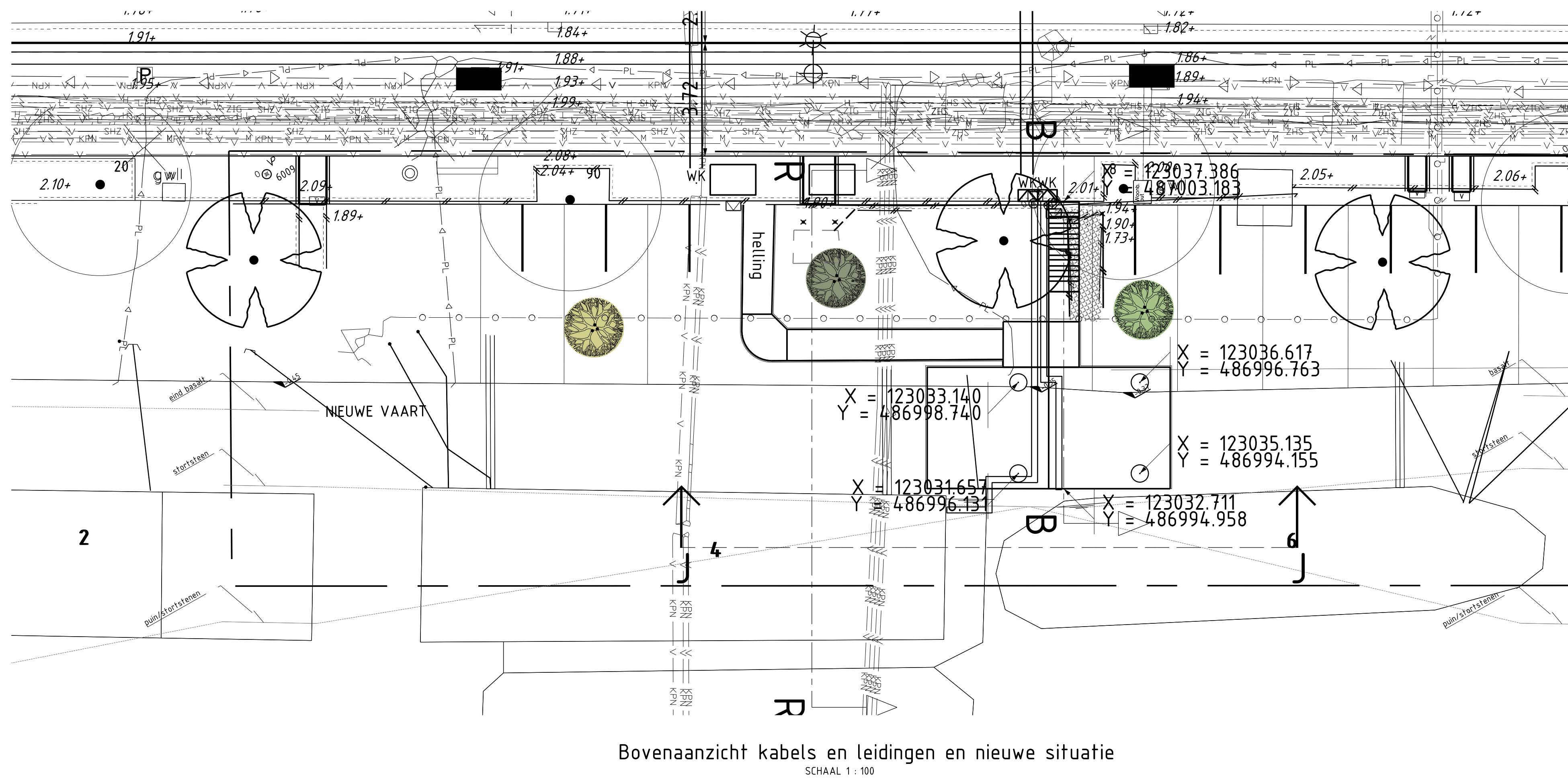
Bovenaanzicht sloopsituatie SCHAAL 1 : 100
