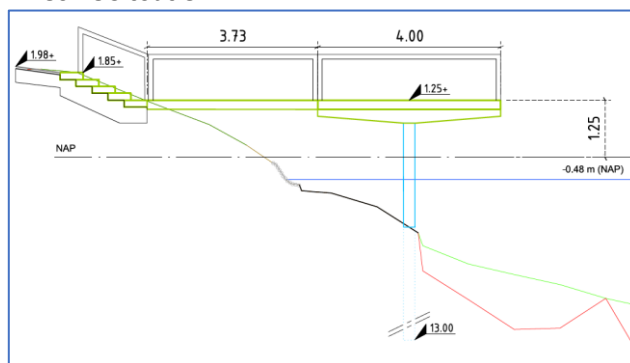
Nieuwe situatie
