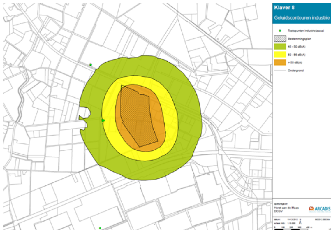
Figuur 13: Geluidscontouren industrie
