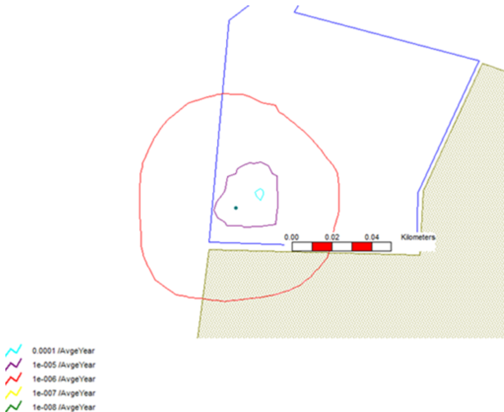
Figuur 14: PR contouren LNG
