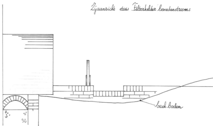
Schaal 1:20
