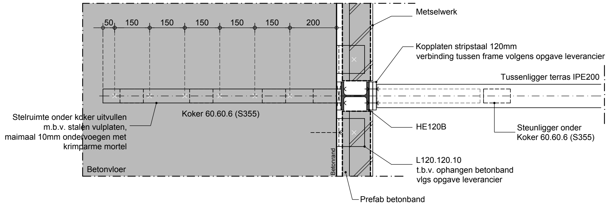
Bovenaanzicht Detail 3 (Constructief)
