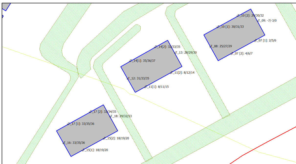
Figuur 5.2: Rekenresultaten vanwege de Vlissingestraat, inclusief aftrek van 5 dB.
